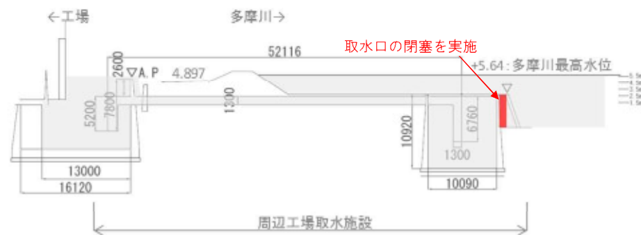
多摩川取水口断面図
