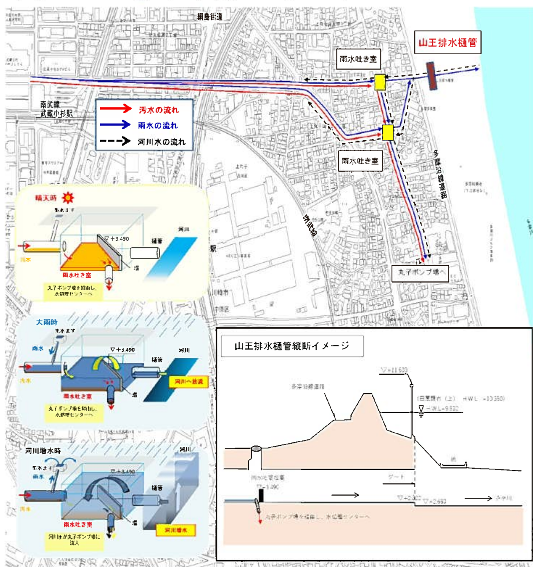
図 3-1-2 丸子その1排水区の雨水吐き室
