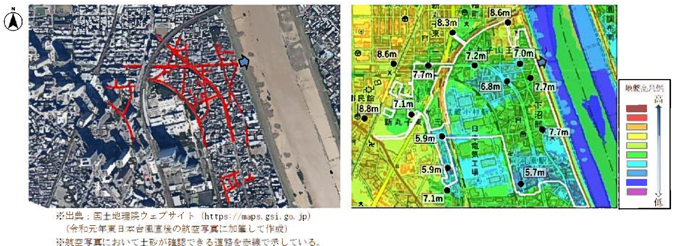
図5-1-2 山王排水樋管周辺の浸水発生区域と地盤高
