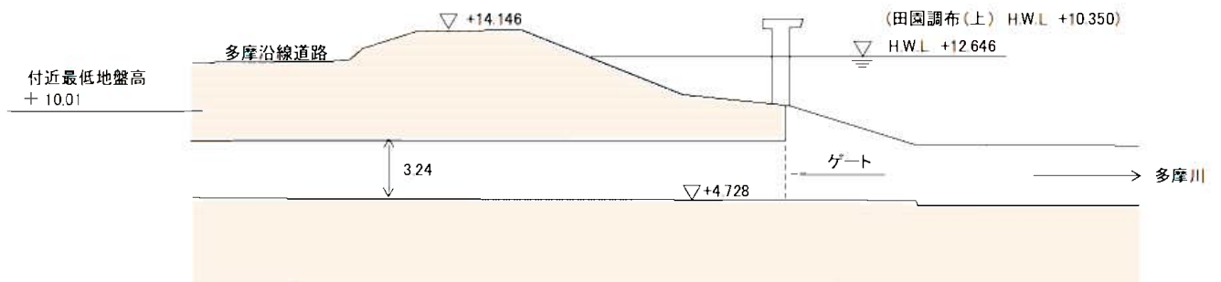
図 4-2-1 宮内排水樋管の概要と縦断面図
