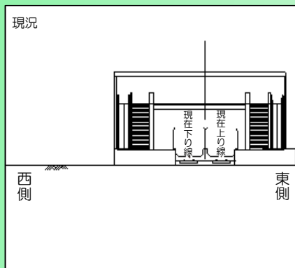
Step1 計画下り線切換
