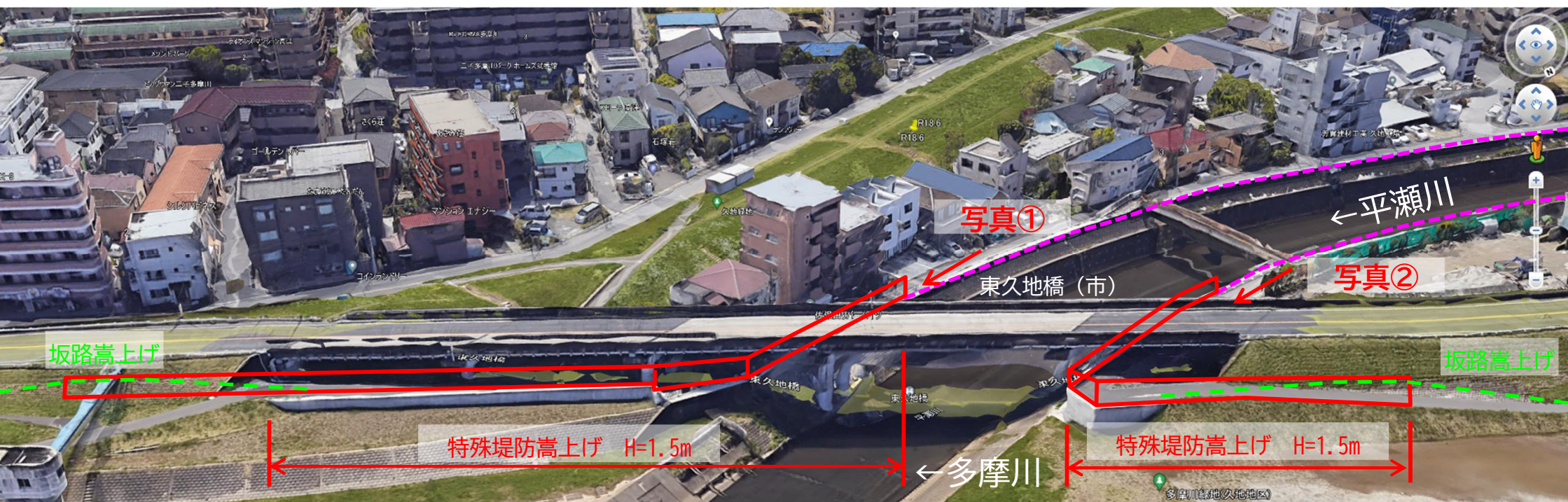
写真①：下流側特殊堤と多摩川河川敷に通じる通路の状況
