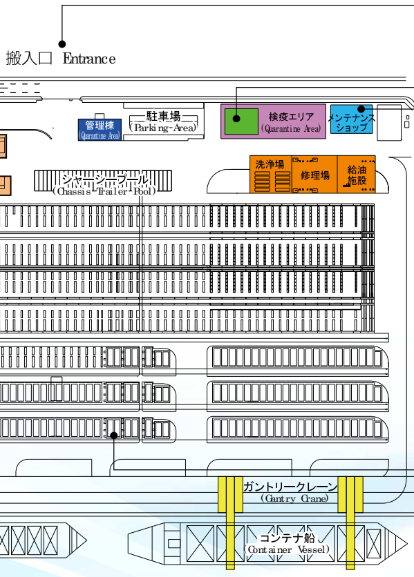
リーファー電源 Power points for a refrigerated container
