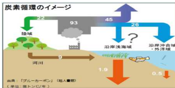
海洋(26億t-C/年)は陸域(22億t-C/年)以上の炭素を吸収 出典：ブルーカーボン研究会「ブルーカーボンについて」 図 ブルーカーボンを活用した炭素循環のイメージ
