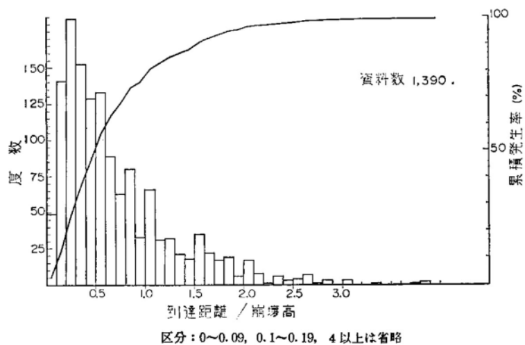
図 5.5-5 降雨による崩壊土砂到達距離と崩壊高の比の度数分布(反町(1978) 15) )
