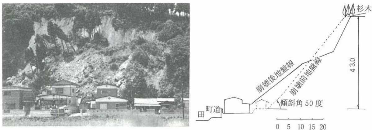
図 5.5-3 1978 年宮城県沖地震 松島町高山下地区がけ崩れ被災状況及び横断図 (土木学会東北支部(1980) 14) )
