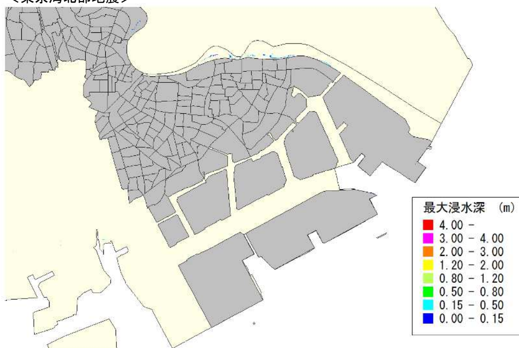
図 5.6-2(2) 津波浸水予範囲 (2) (第3編 編末図-2を再掲)
