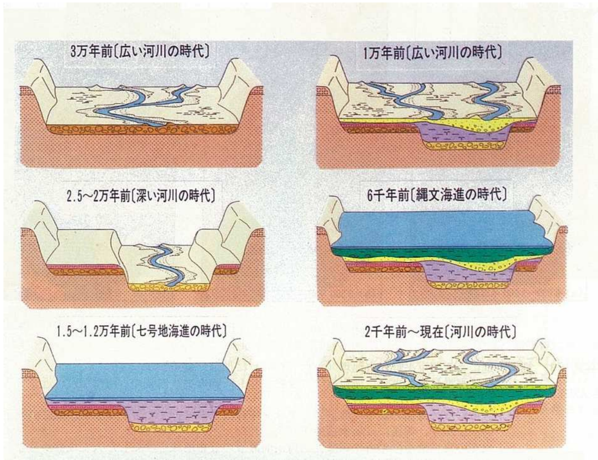
図1 沖積層の形成モデル
