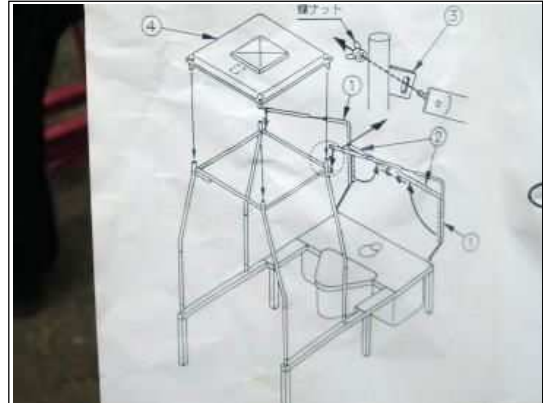
③-1 天蓋の組立図
