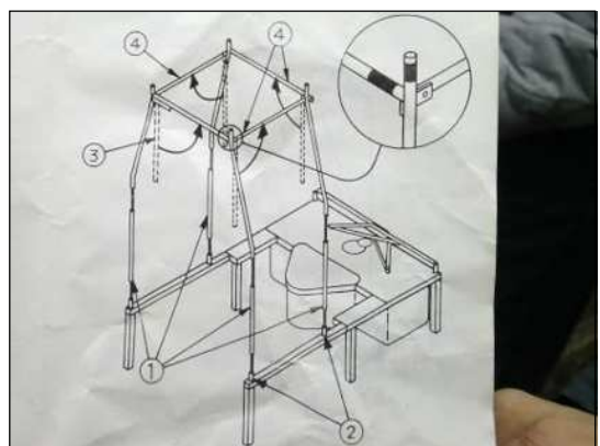
②-1 支柱の組立図
