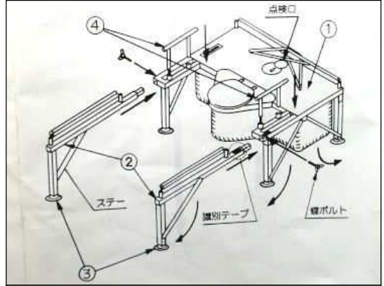
①-3 架台の組立図
