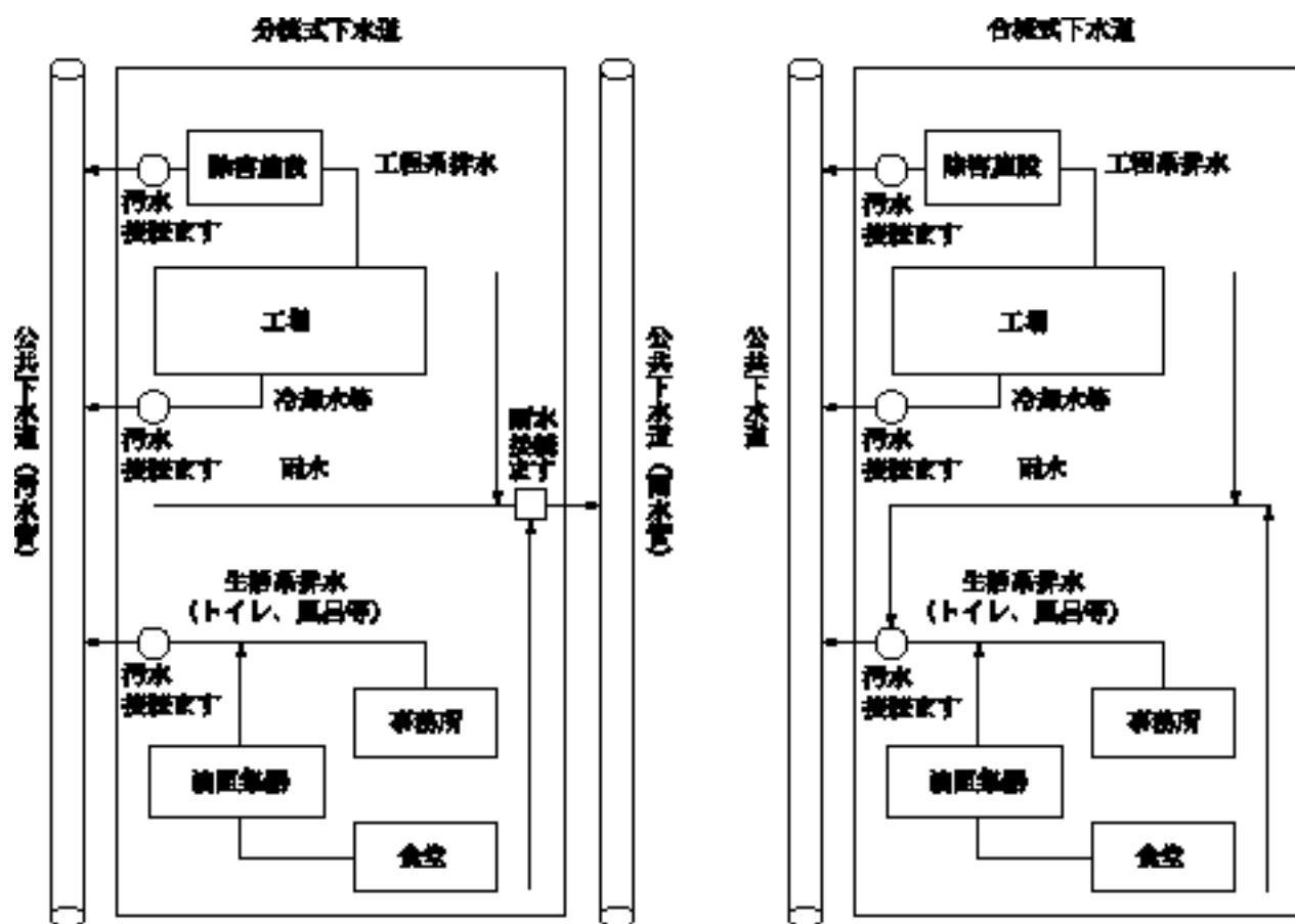
図 2－2 排水系統の例
