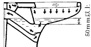
図 2-19 ブローアウト式
