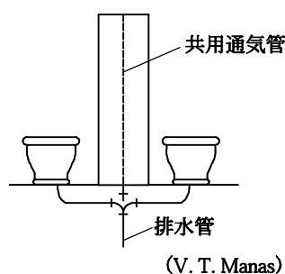
図2-31 共用通気にできる場合の例
