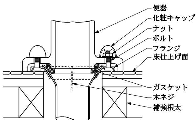
図 2-22 洋風大便器の施工例 (ロータンク式)
