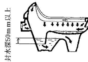
図 2-15 洗出し式
