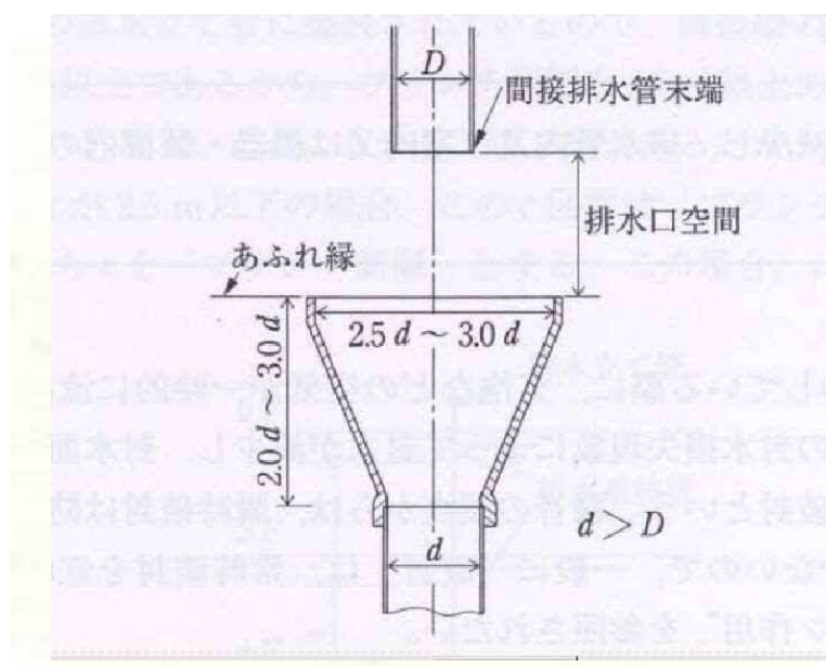
図 2-4 2 排水口空間
