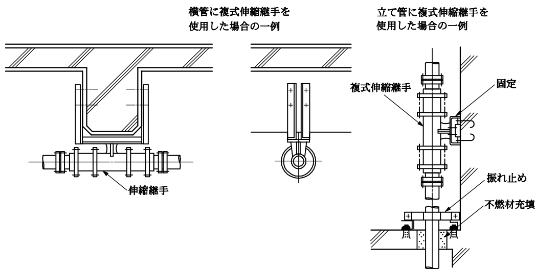
図 2－3 管の損傷防止措置例
