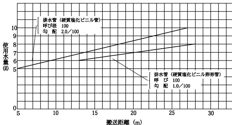
図2-21 使用水量による搬送距離
