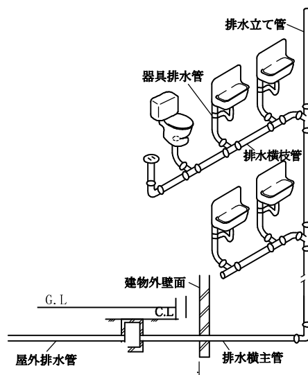
図2-1 排水管の種類
