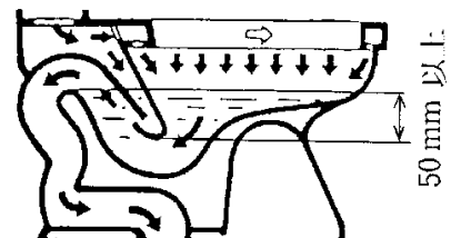
図 2-17 サイホン式
