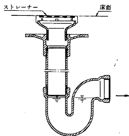
図 2-12 床排水トラップの例
