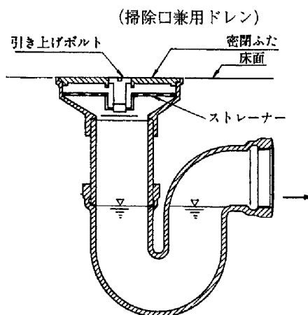
図 2-13 床排水トラップの例
