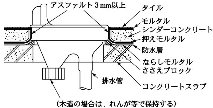
図 2-23 和風大便器の施工例
