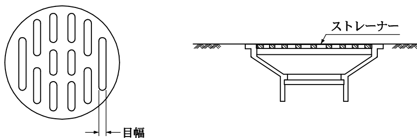
図2-43 ストレーナーの例(目皿)
