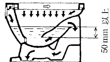
図 2-17 サイホン式
