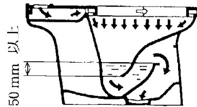
図 2-16 洗落とし式
