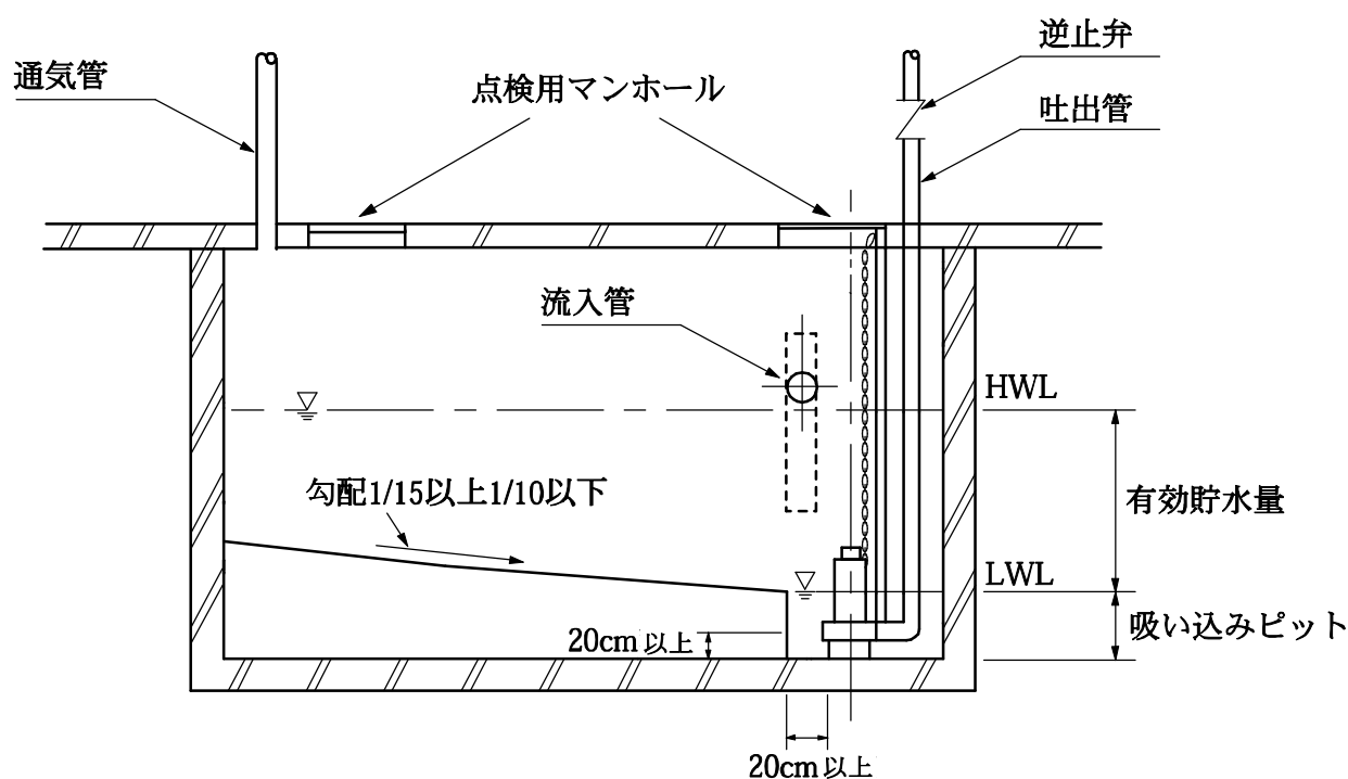
図 2—4 1 排水槽の例
