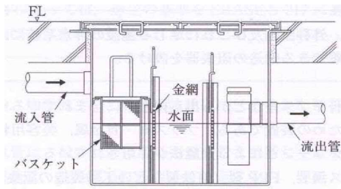
図 2－39 繊維くず阻集器の例
