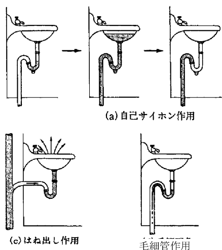
図 2-10 トラップ封水の破られる原因
