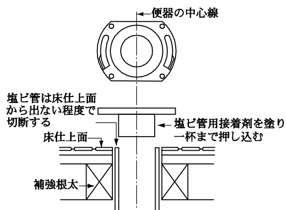
図 2-22 洋風大便器の施工例 (ロータンク式)
