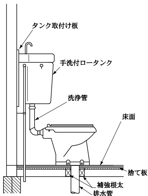
(b) 排水管が硬質塩化ビニル管の場合
