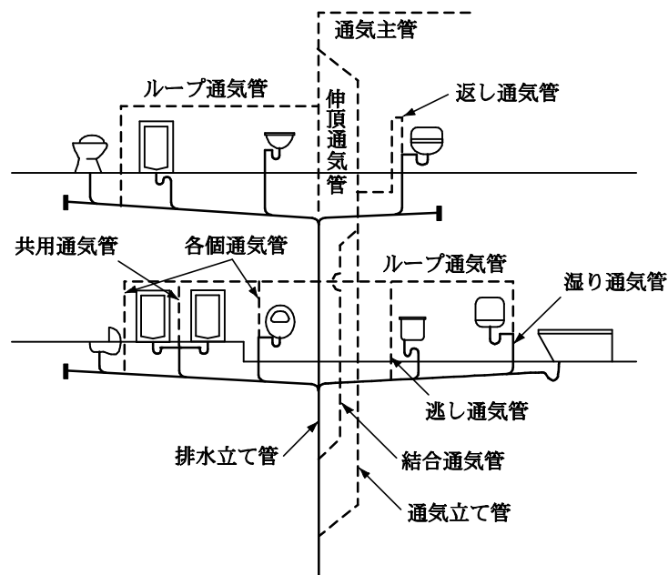
図 2-24 各種通気管の種類
