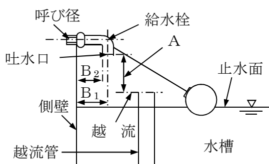
図 1-4 越流管
