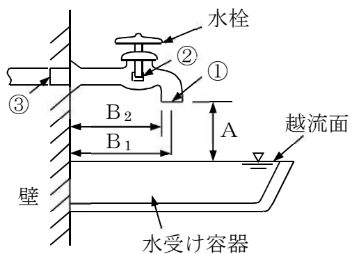
図 1-3 水受け容器
