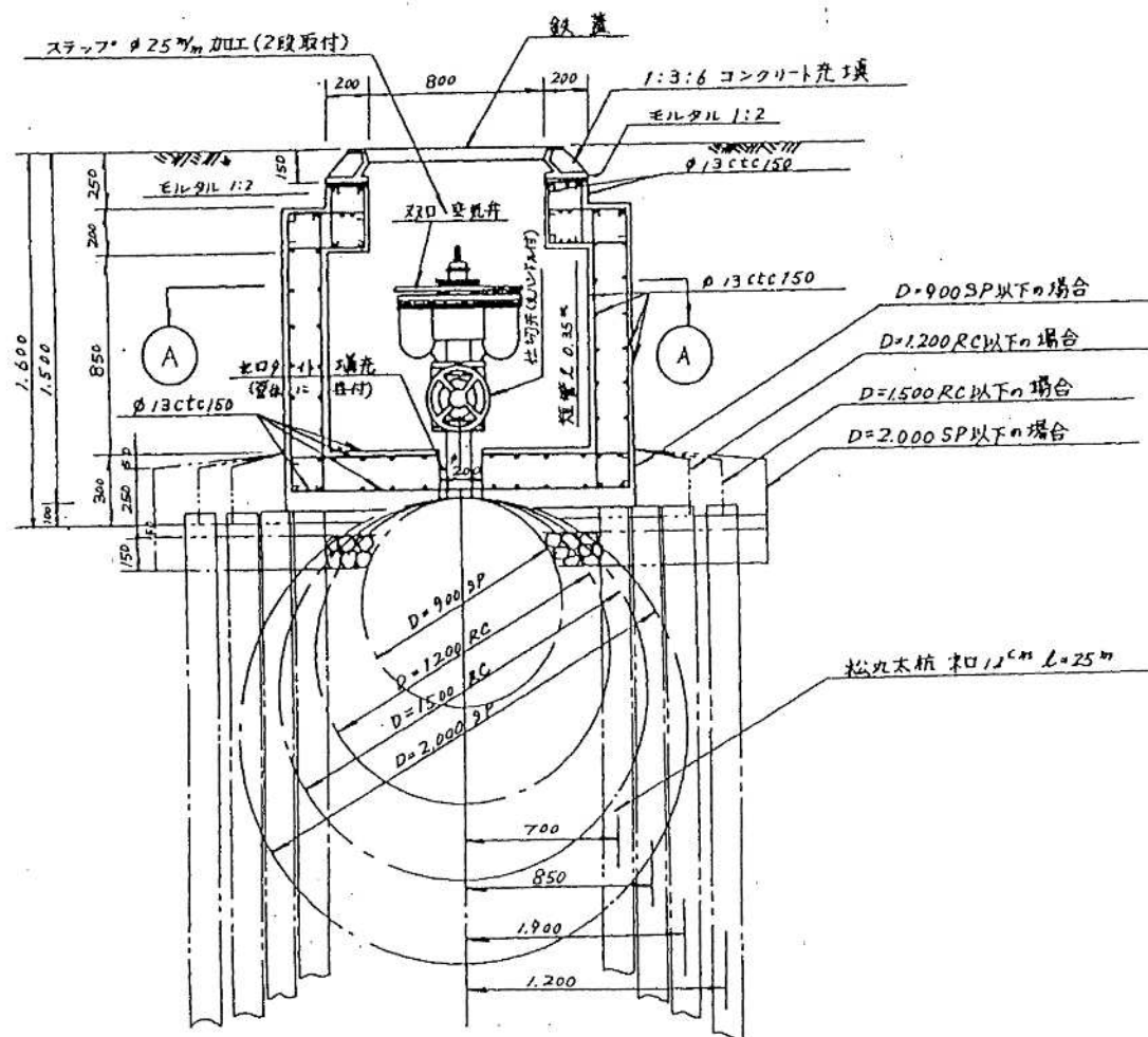
空気弁室設置図断面図 S = \frac{1}{20}
