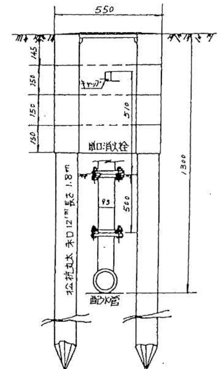
② - ② 断面図
