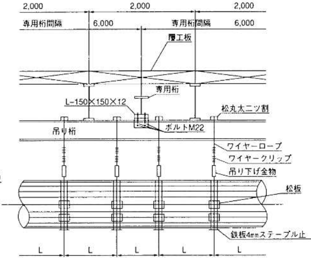
側面図
