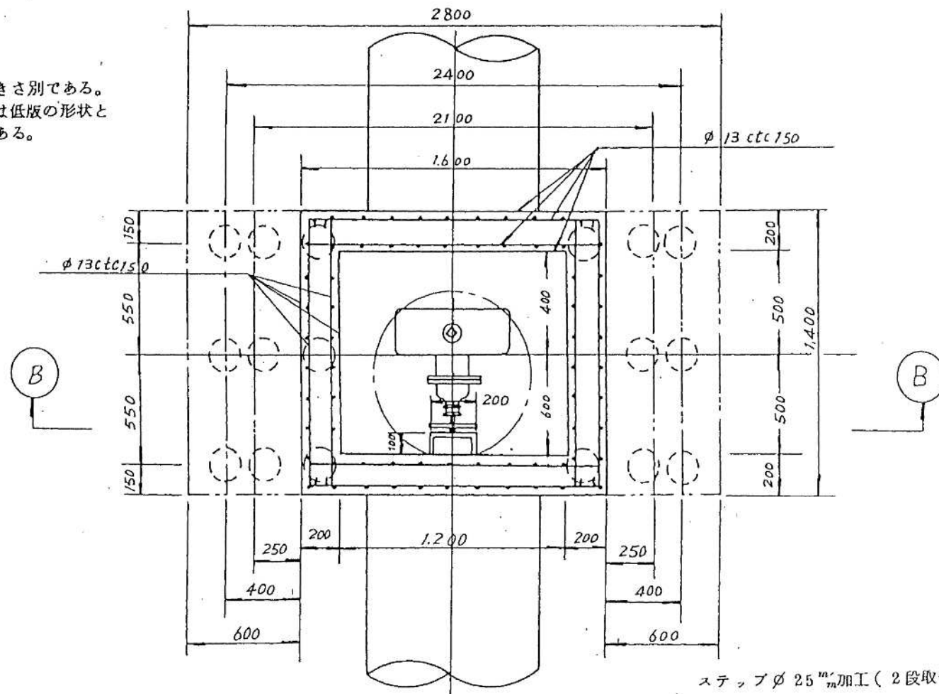
空気弁室設置図(平面図1) S = 1\frac{1}{2}0
