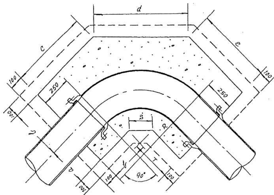
90° 曲管防護図 ( 水平 )
