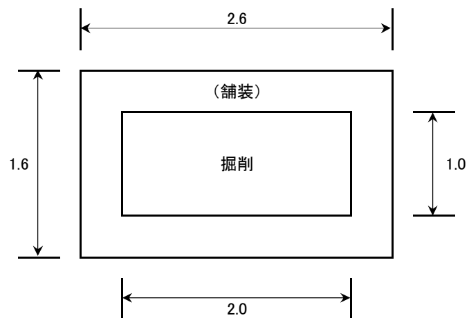
平面図
