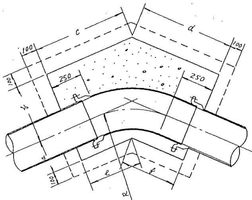
45°曲管防護図（水平）
