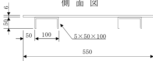
側面図
