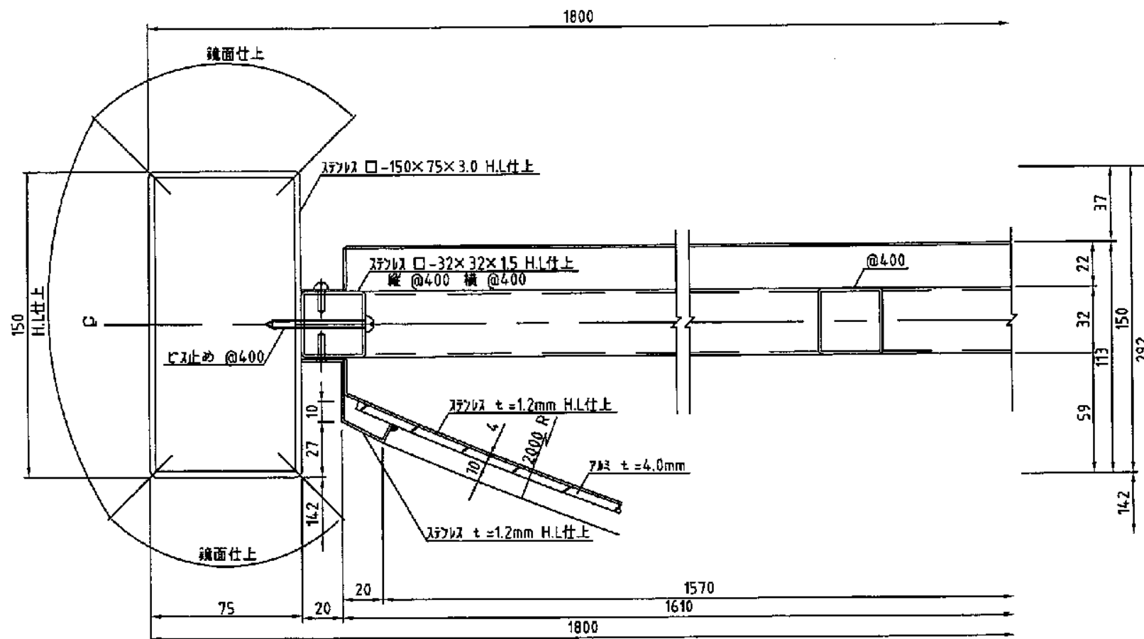
平 断 面 図
