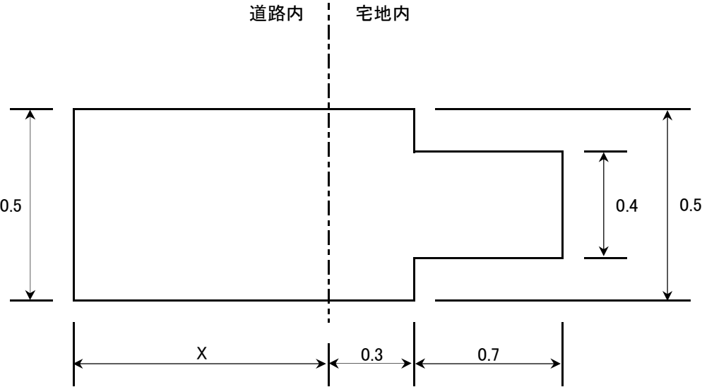
横断面図
