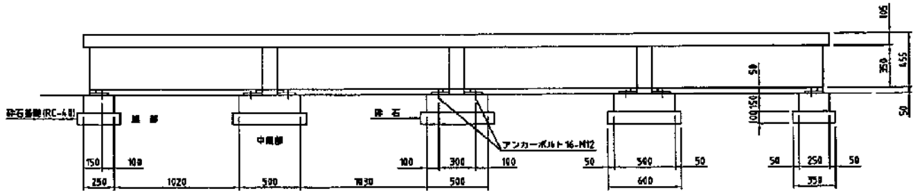
断面図
