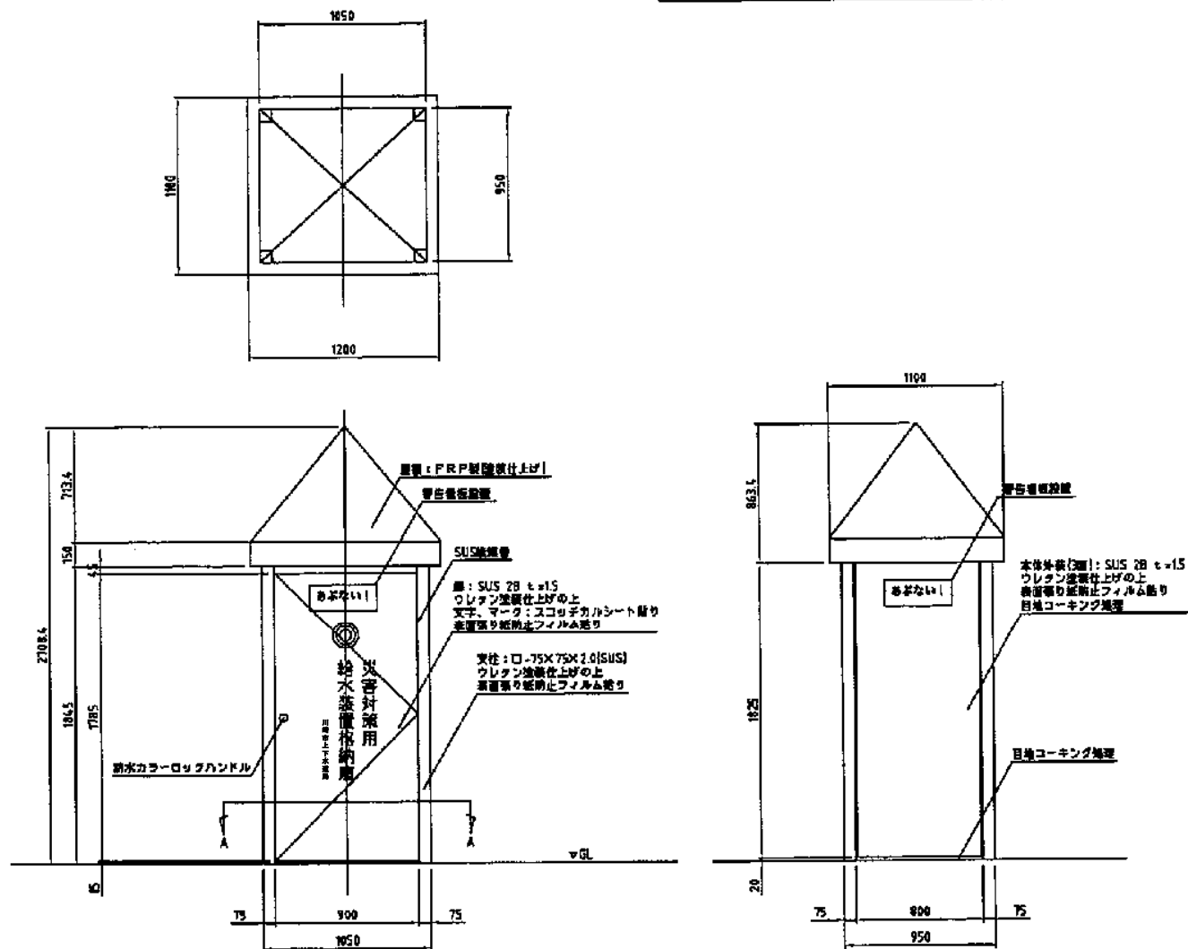
手押しポンプ用格納庫製作図
