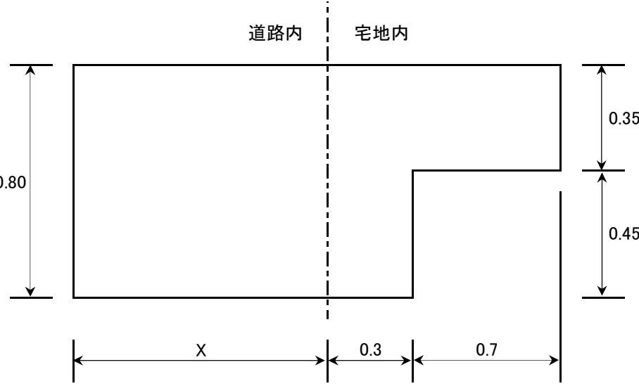
横断面図
