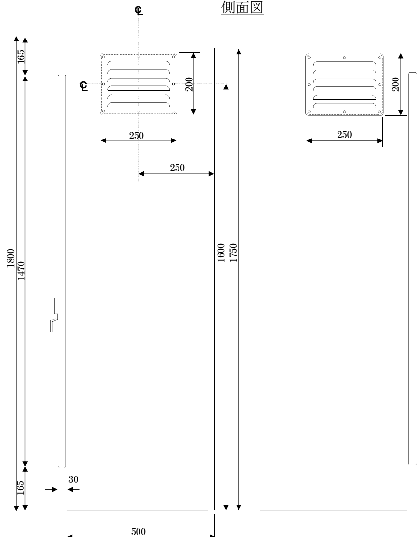
側面図
