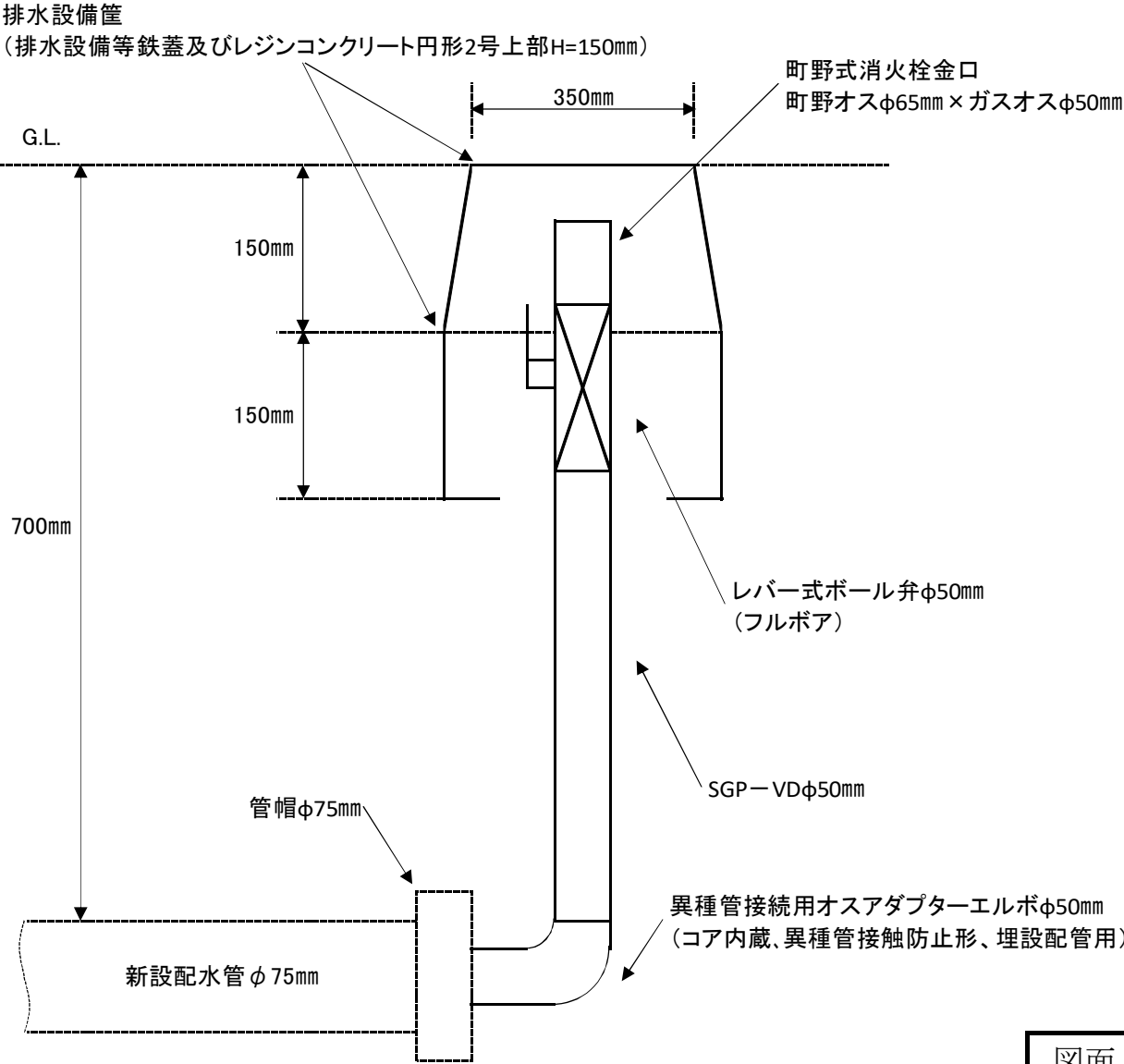
簡易排水設備設置標準図
