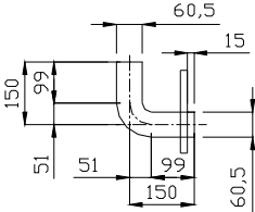
空気抜き50A 詳細図
