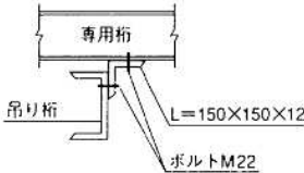
吊り桁取付詳細図
