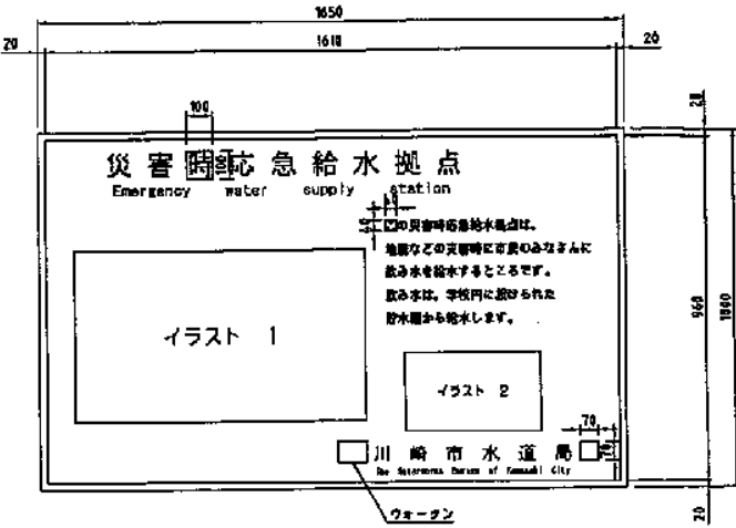
標示板寸法図 縮尺=1/20
