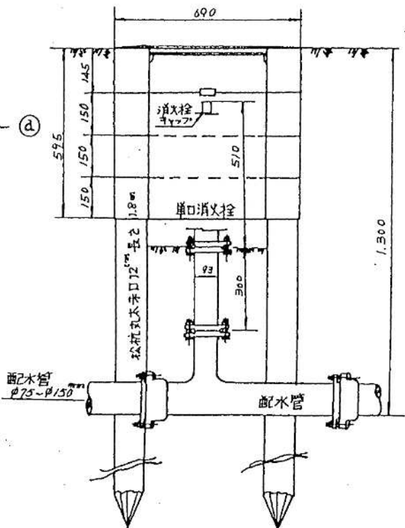
① - ① 断面図 S = 1 : 10
