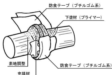
図 1-17 接合部充てん、防食テープ巻き参考図
