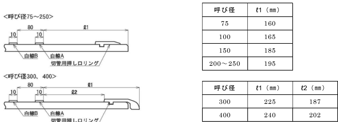
図 1 - 8 挿口加工図及び寸法
