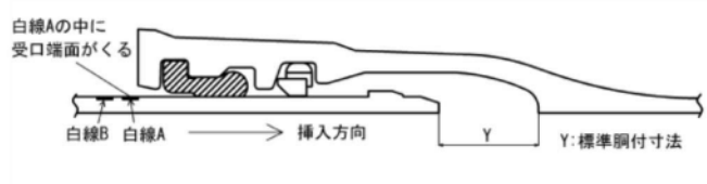
図 1-7 接合状態図
