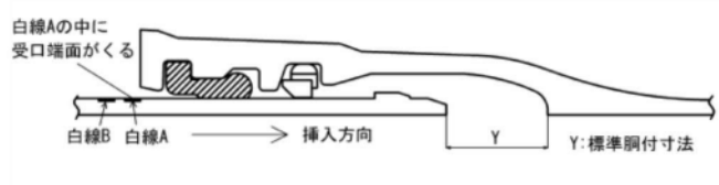
図 1-7 接合状態図
