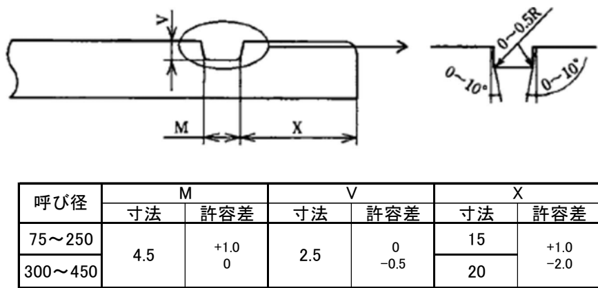
図 1 - 11 挿口加工図及び寸法
