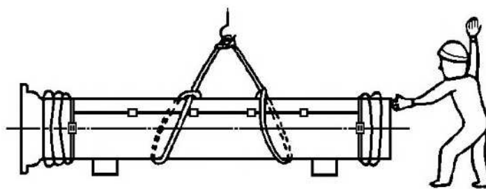
図 1 - 2 吊り方の例
