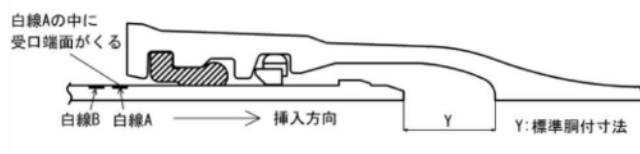
図 1-7 接合状態図
