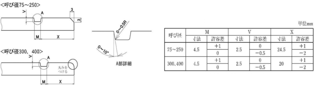
図 1－8 挿口加工図及び寸法
