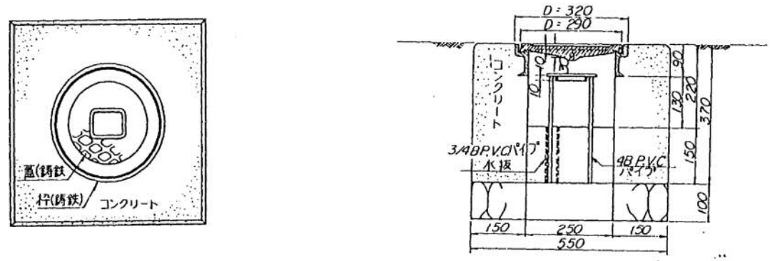
電気防蝕用ターミナル(排流点兼用)
