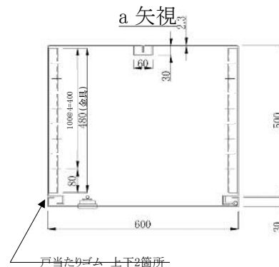
金具 (フック設置時)
