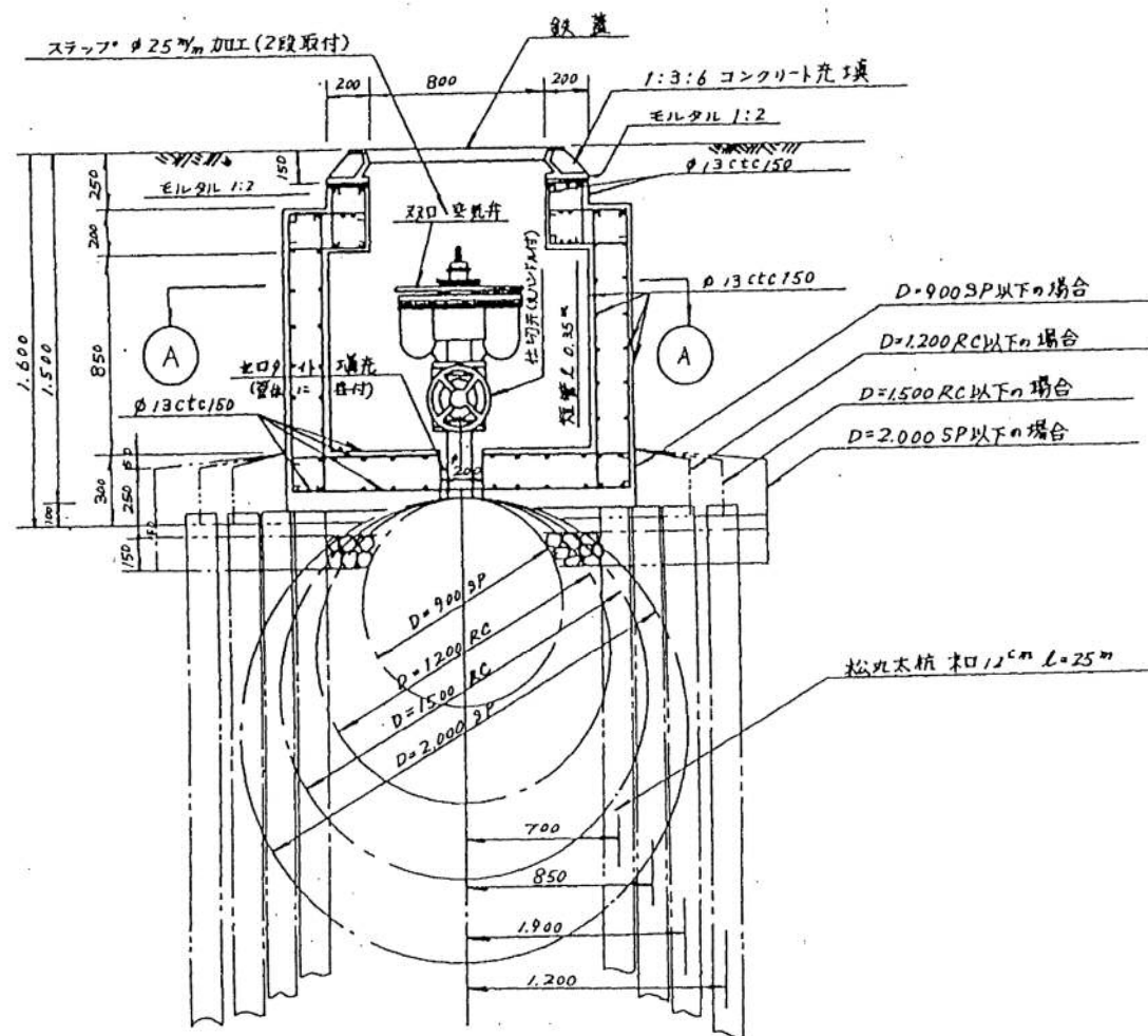
空氣弁室設置図断面図 S = \frac{1}{20}
