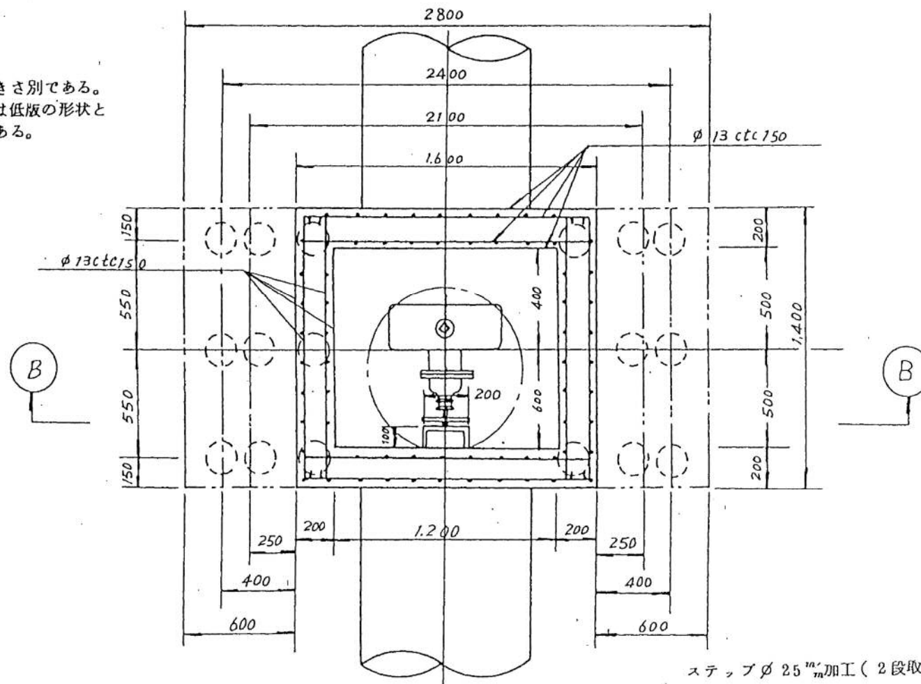
空気弁室設置図(平面図1) S = 1\frac{1}{2}0
