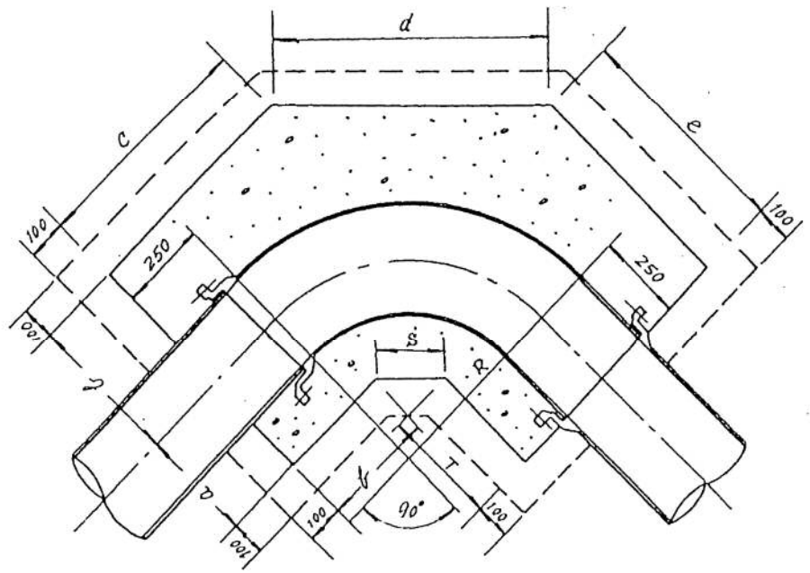
90° 曲管防護図 ( 水平 )
