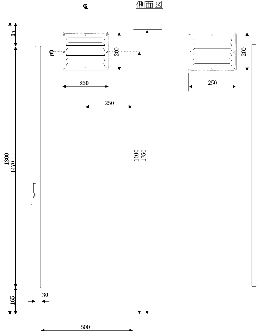
側面図
