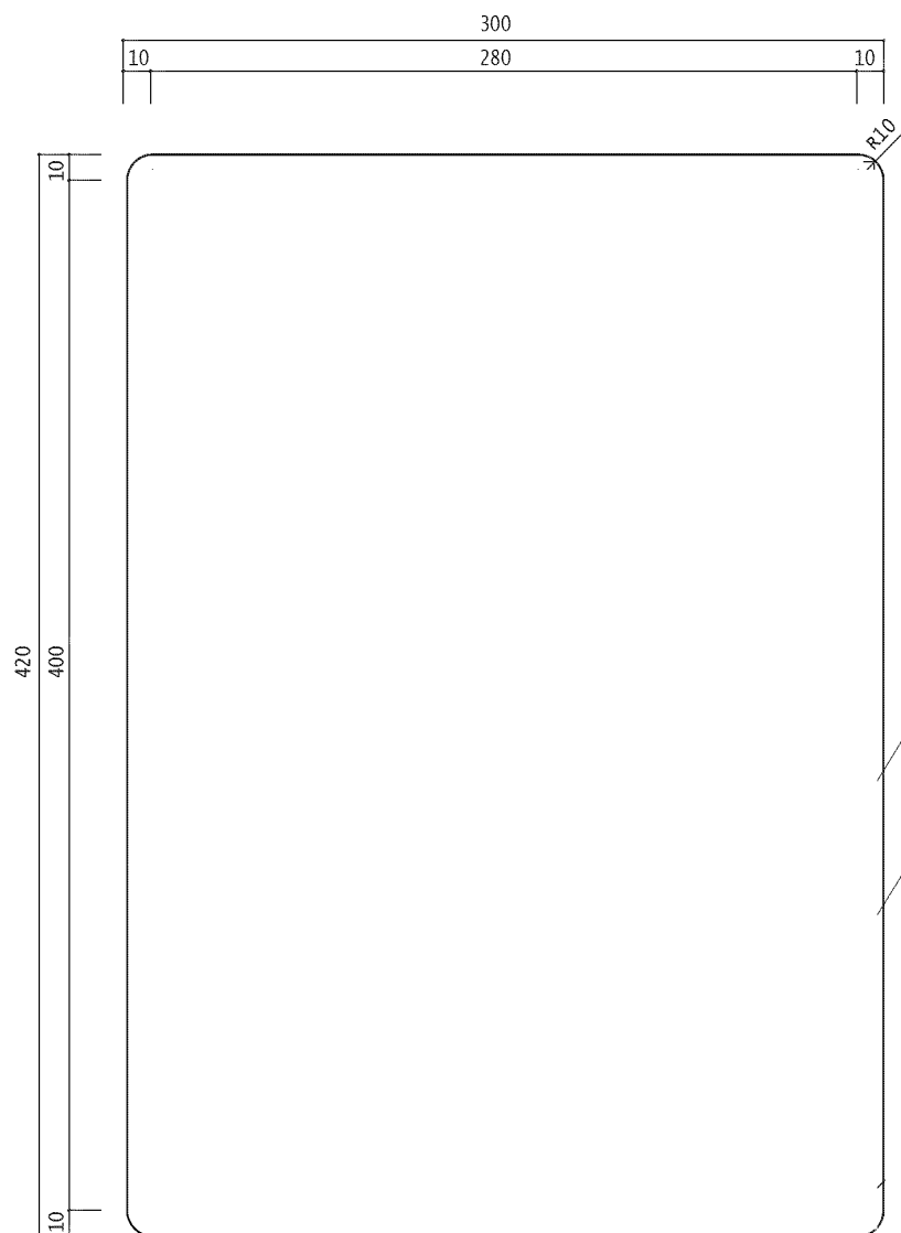
平 面 図
