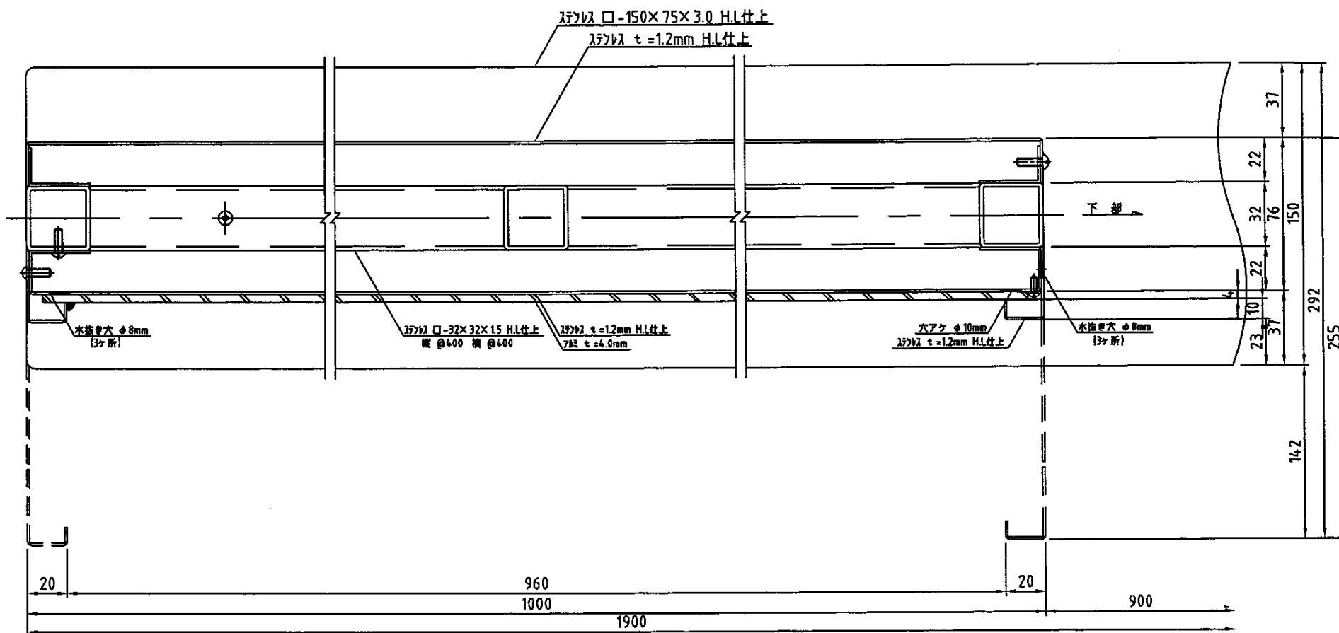
立断面図
