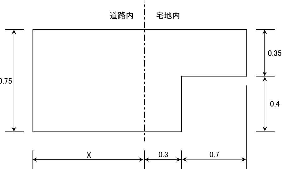
断面図
