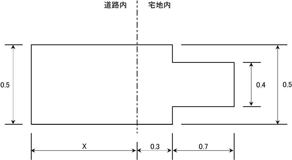
断面図
