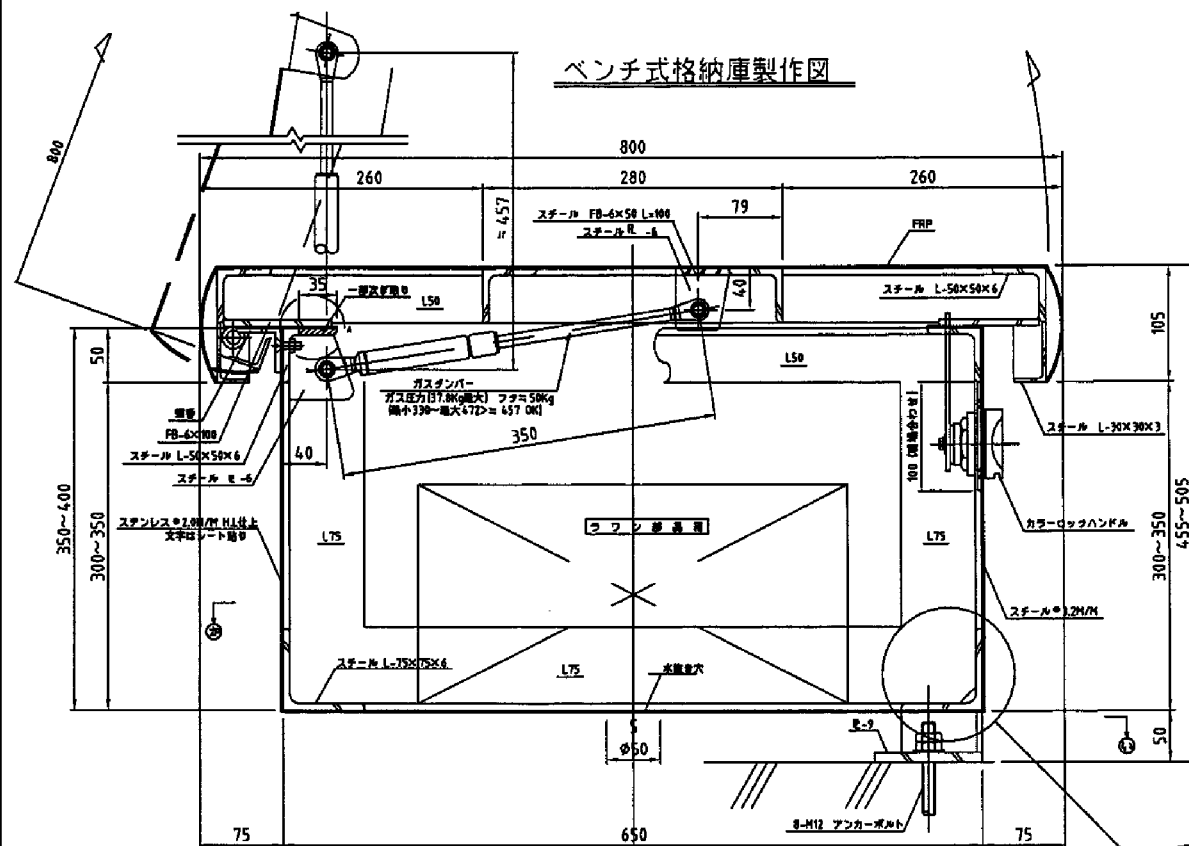
① 正面図
