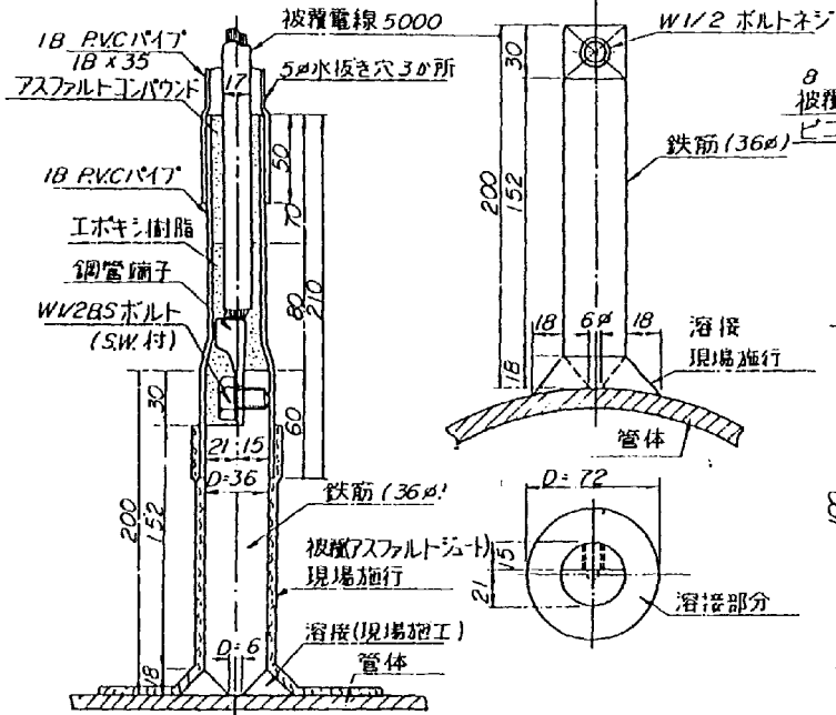
電気防蝕用ターミナル(排流点兼用)
