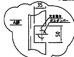
② 側面図
