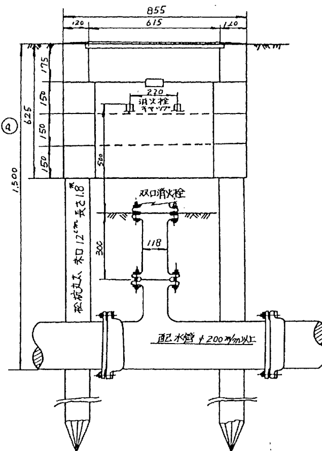
① — ① 断面图
