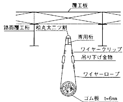
内径350未満断面図
