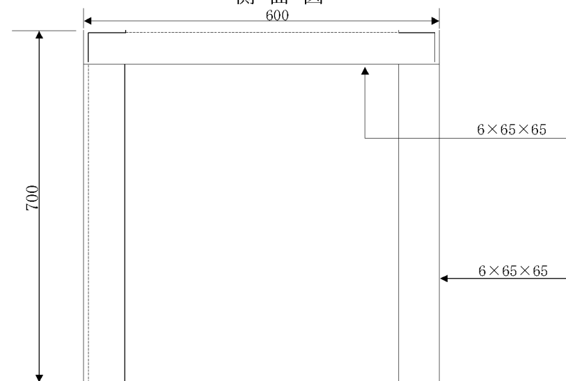
側面図
