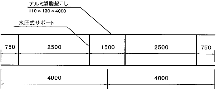
支保工設置図
