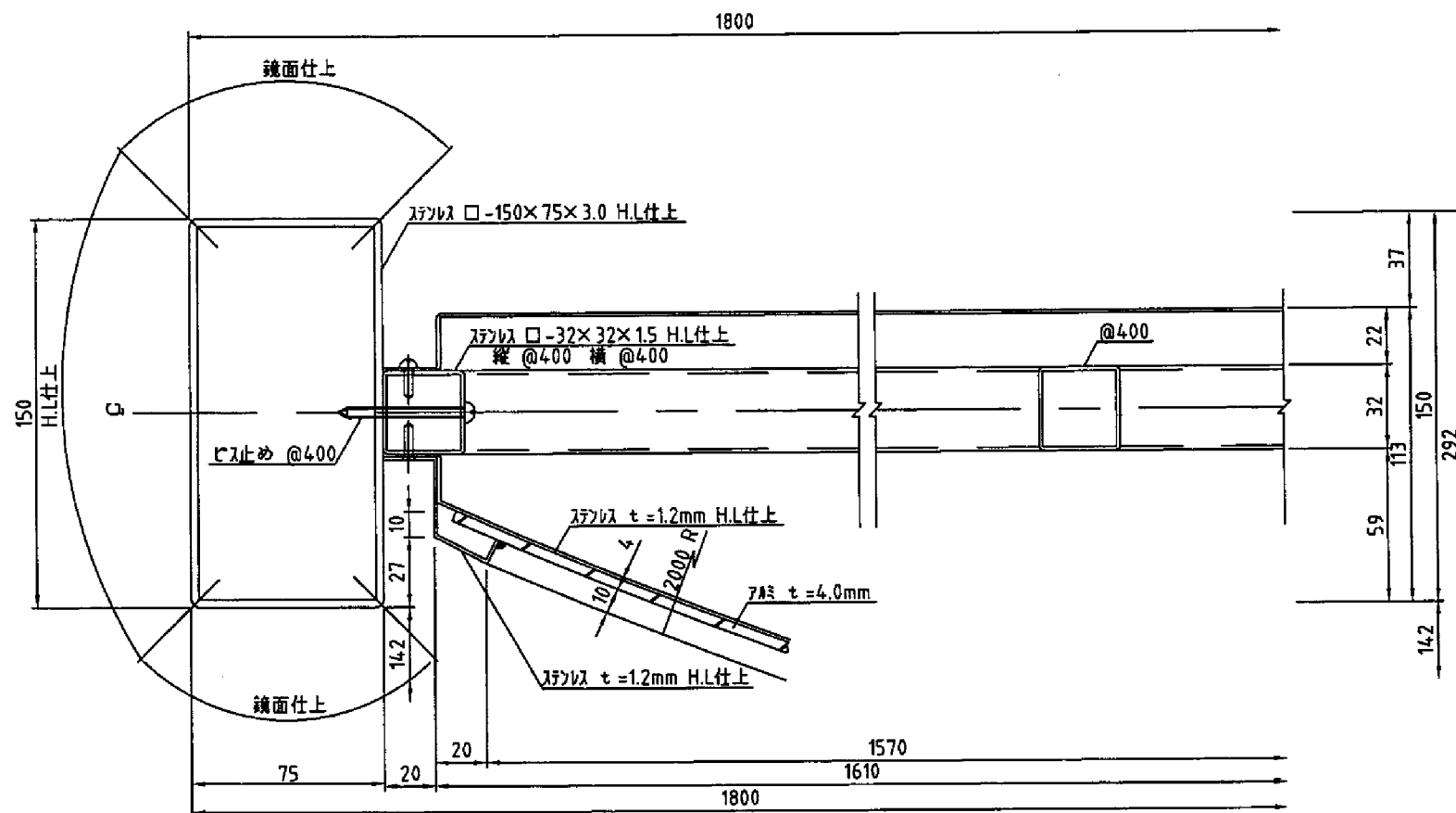
平 断 面 図
