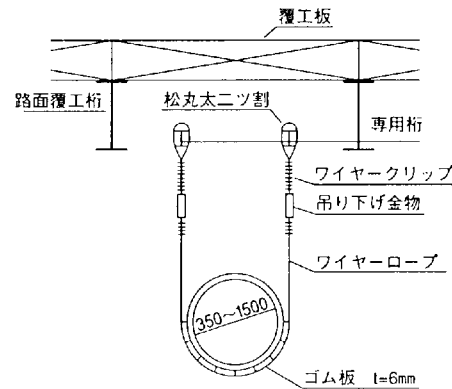
内径350以上断面図
