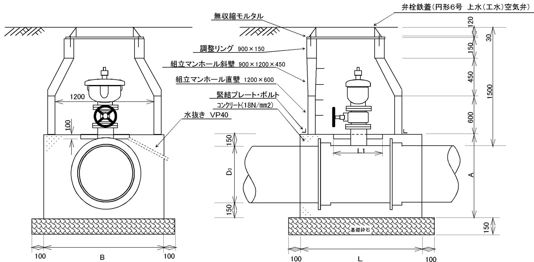
寸法表
