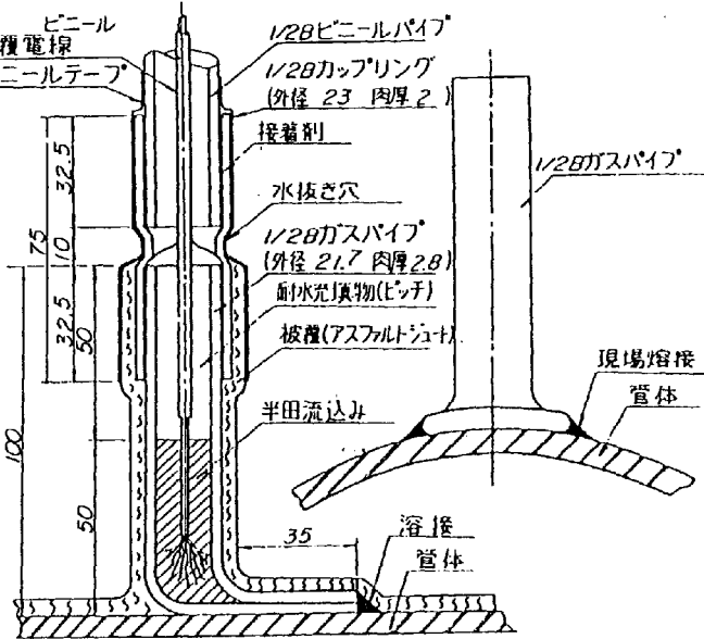
電気防蝕用ターミナル(電位測定用)
