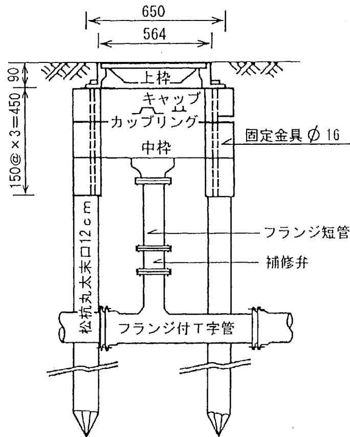
① - ① 断面図
