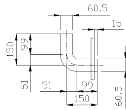
空気抜き50A 詳細図
