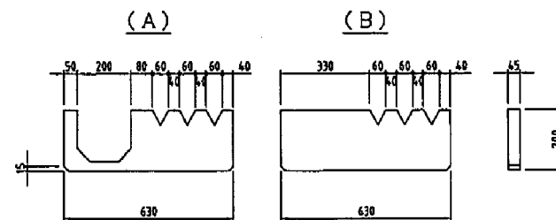
枕 木
