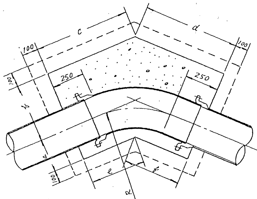
45°曲管防護図（水平）
