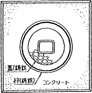
電気防蝕用ターミナル(排流点兼用)
