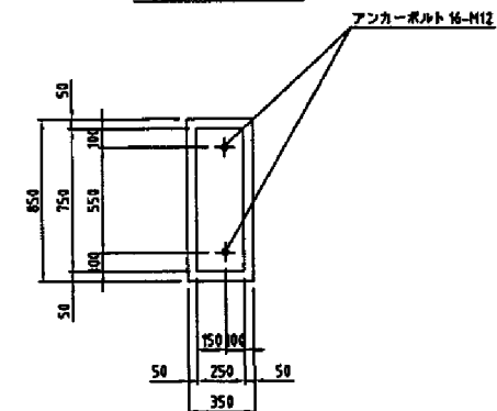
端部
