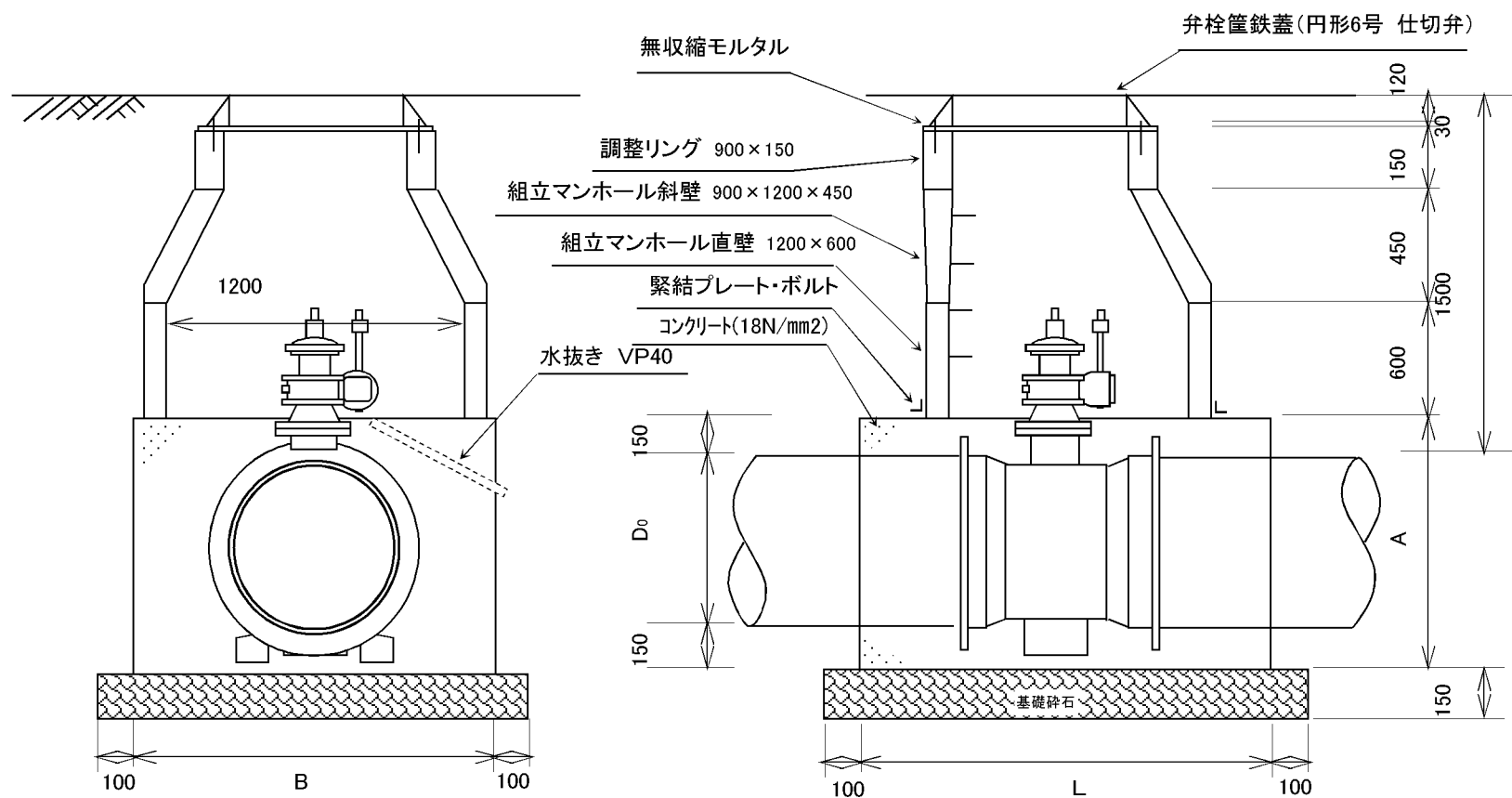
寸法表
