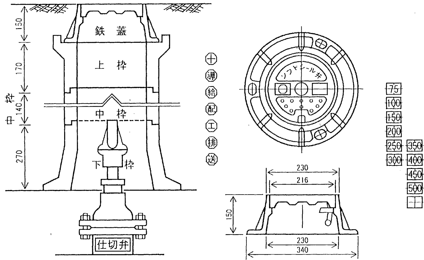
◎浅層埋設
