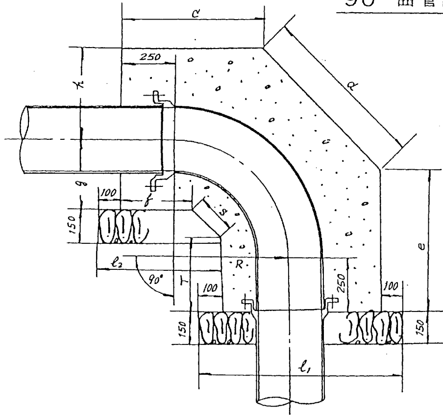
90° 曲管防護図 (垂直)
