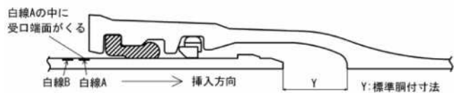
図 1-7 接合状態図
