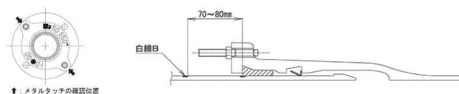
図 1-14 締付け完了状態図
