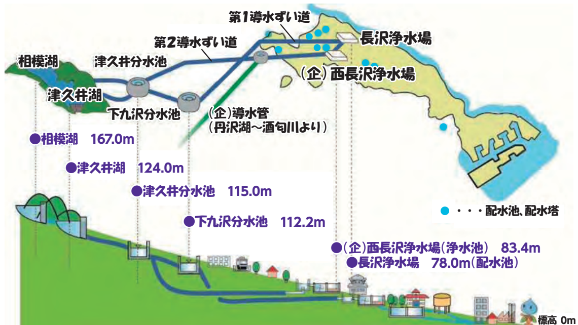
自然流下による水道システム
