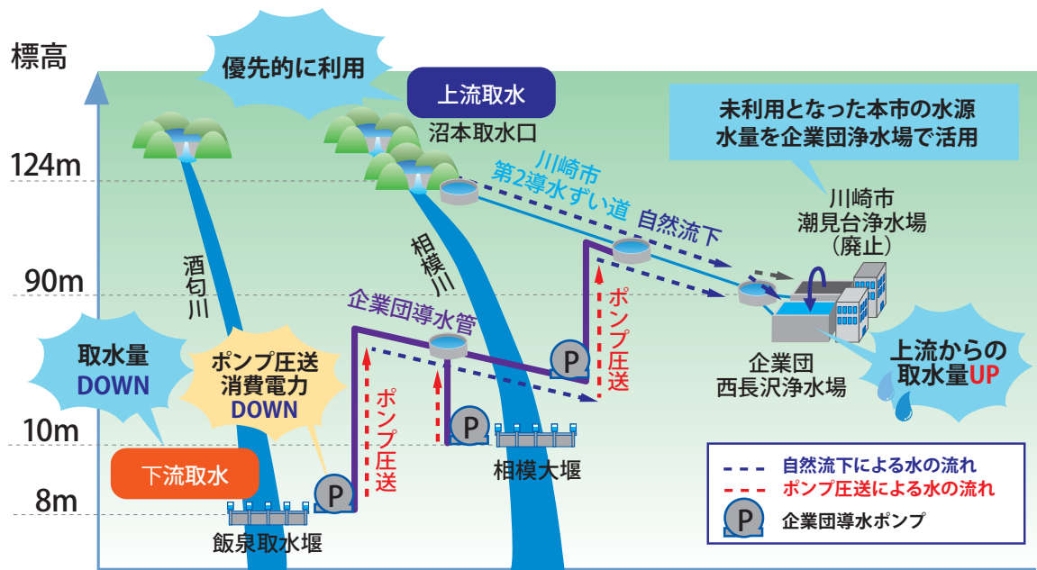
上流取水の優先的利用（イメージ）
