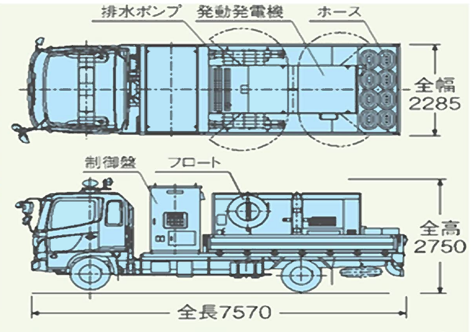
外形図
