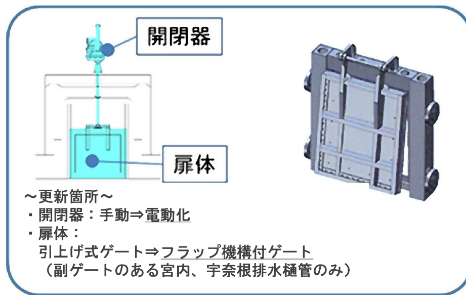
ゲートの改良イメージ
