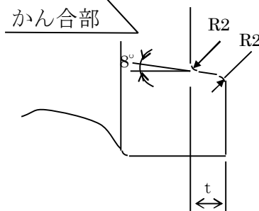
かん合部詳細図
