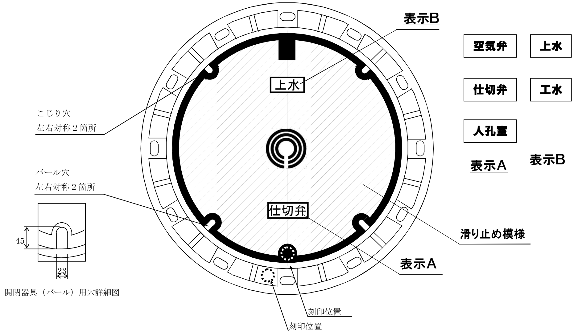
図4 空気弁等鉄蓋（6号（900））表示
