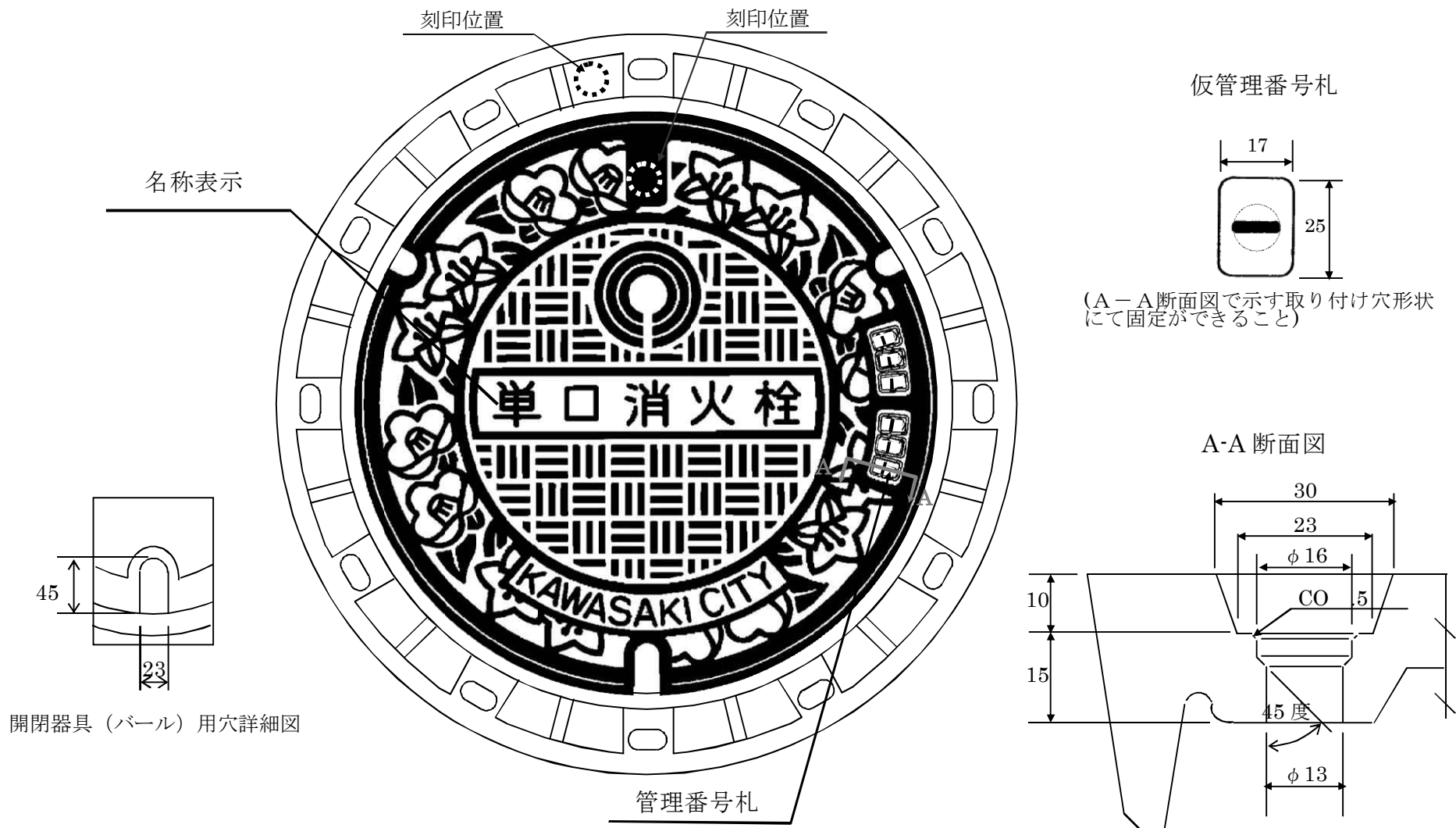
図 3 - 1 消火栓・空気弁鉄蓋・排水弁・仕切弁（3号（500）、4号（600））表示
