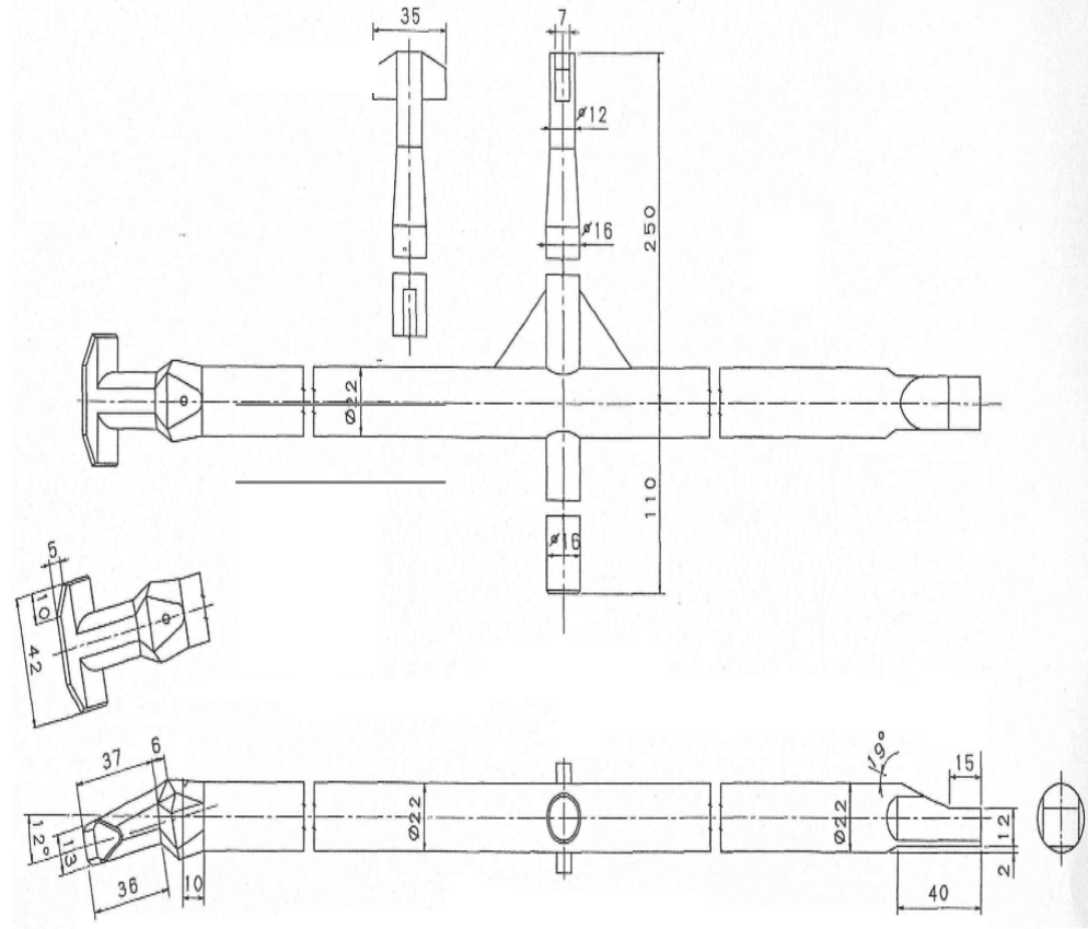
図 6 専用開閉器具（ボール）参考図
