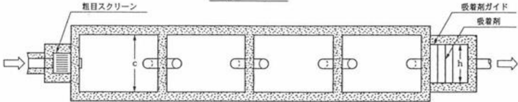
平面
