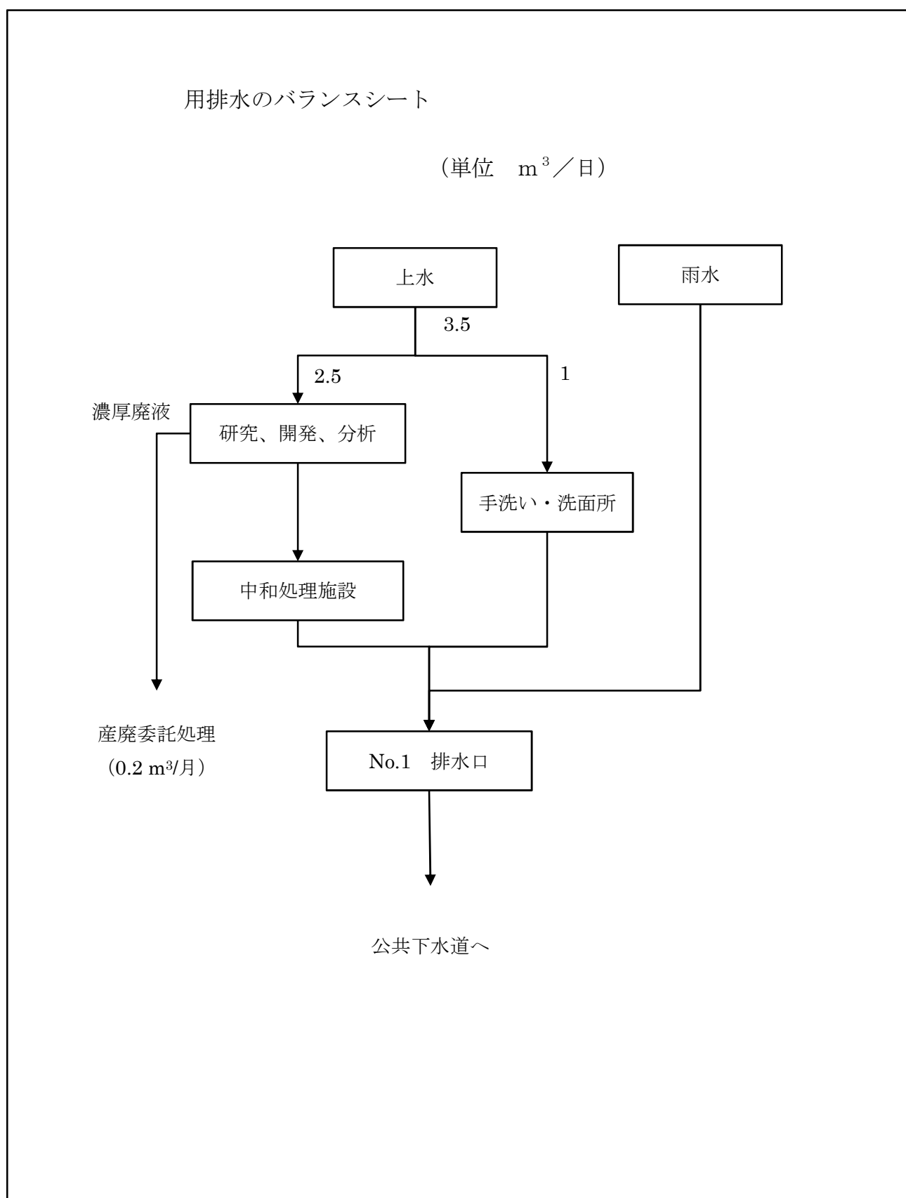
添付表 - 1 用排水のバランスシートの例
