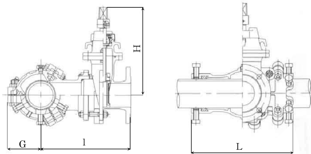
同口径用仕切弁付割 T 字管
