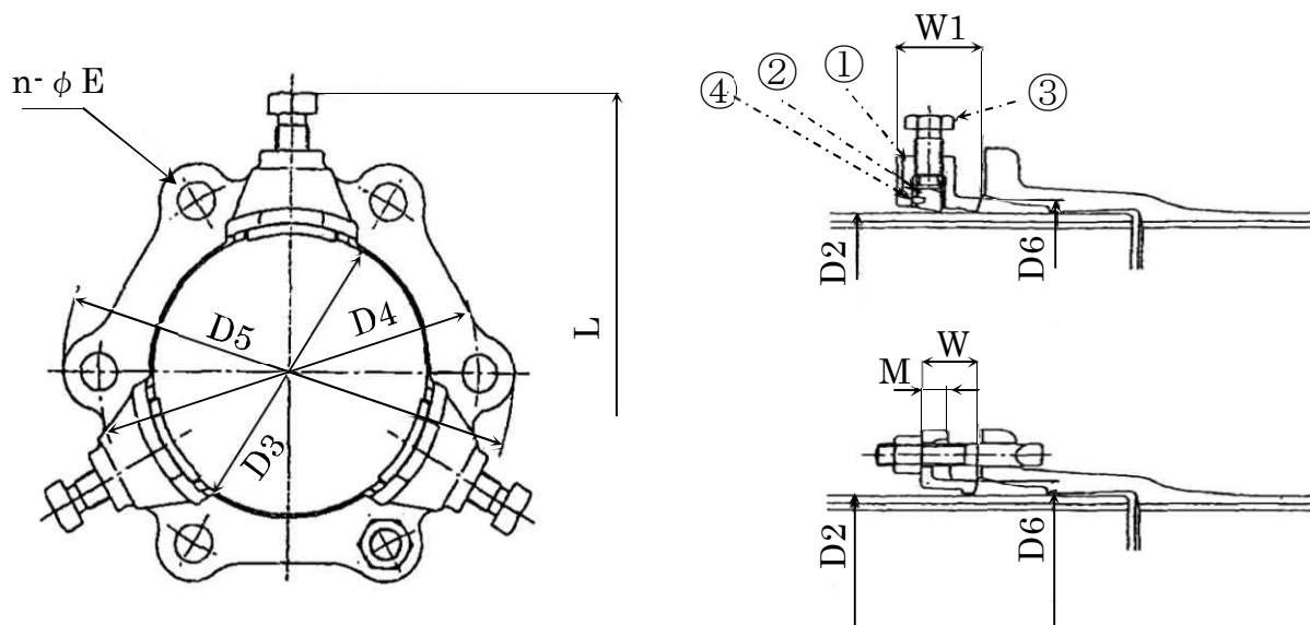
離脱防止押輪の寸法
