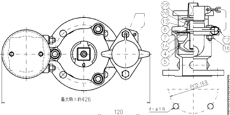
参考図 空気弁付単口消火栓-1
