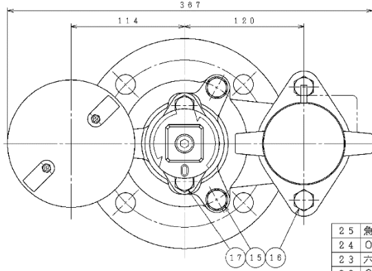
参考図 空気弁付単口消火栓-2. 1
