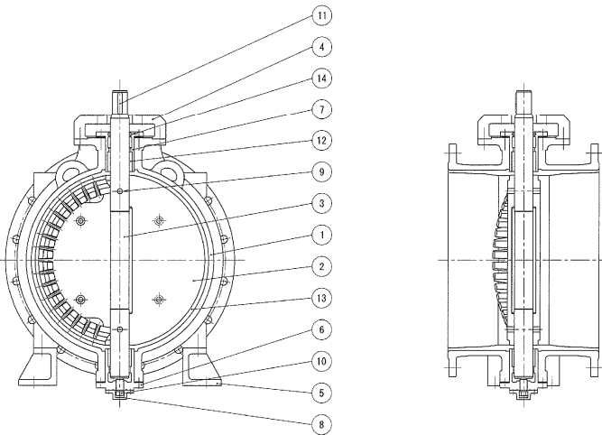
NS 形充水機能付バタフライ弁 参考図③-2 (\phi 500 操作機図)
