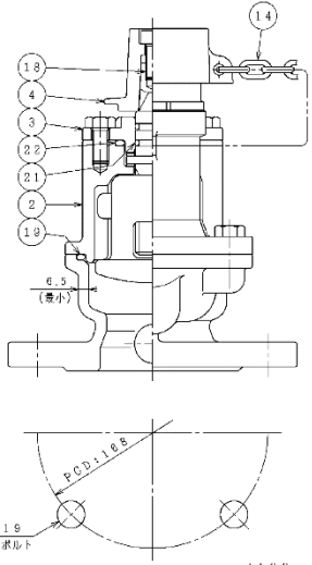
参考図 空気弁付単口消火栓-2. 1
