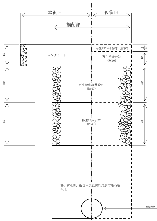
コンクリート舗装（15cm）
