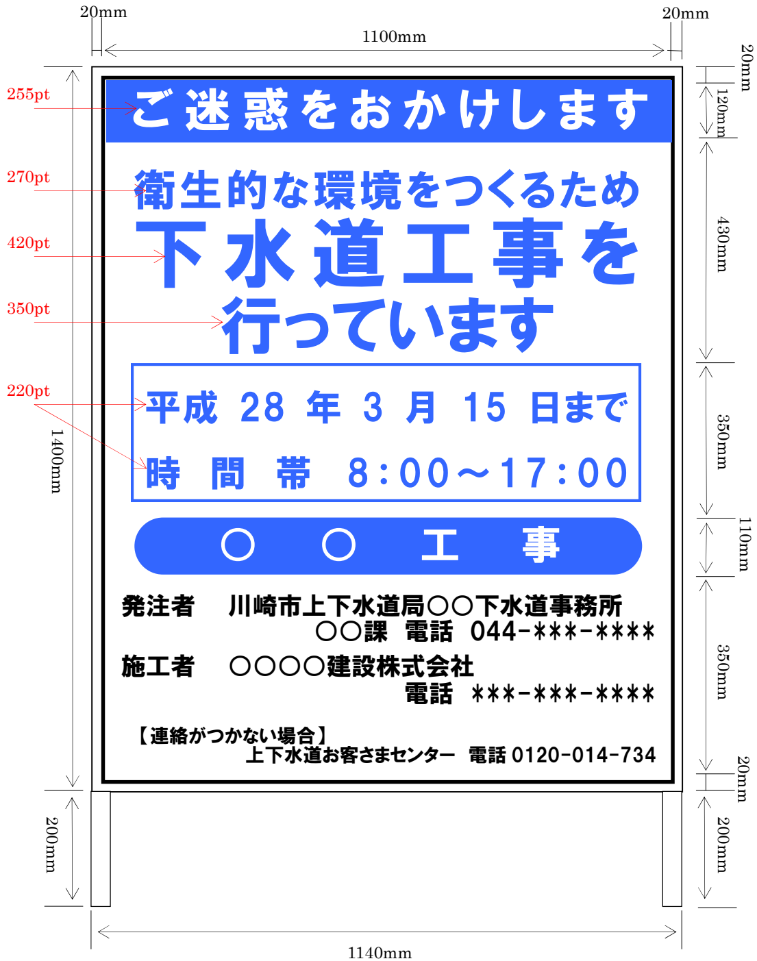
図-1 ①工事中標示板の標準様式
