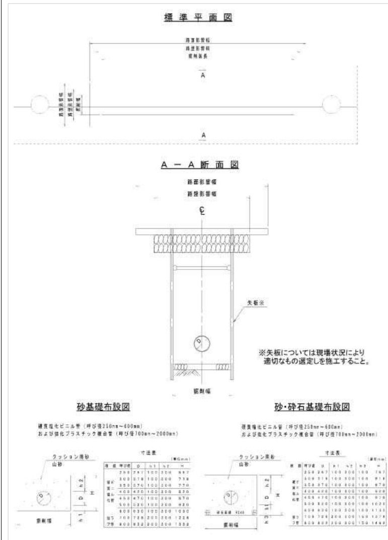
附則ー4 本管施工標準図
