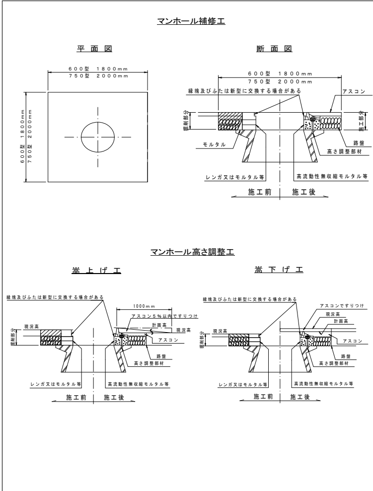
附則－6 マンホール施工標準図
