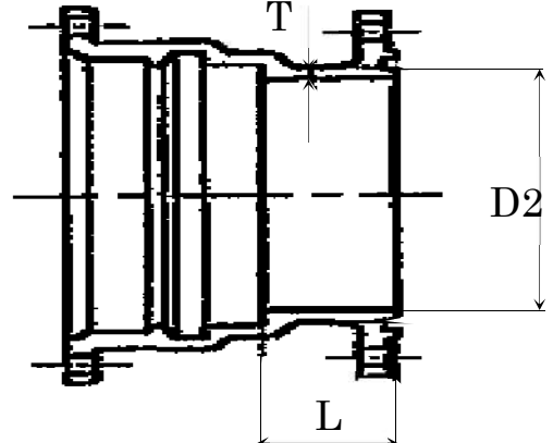
短管 1 号 (φ 300~400) 【10K】 GF 形
