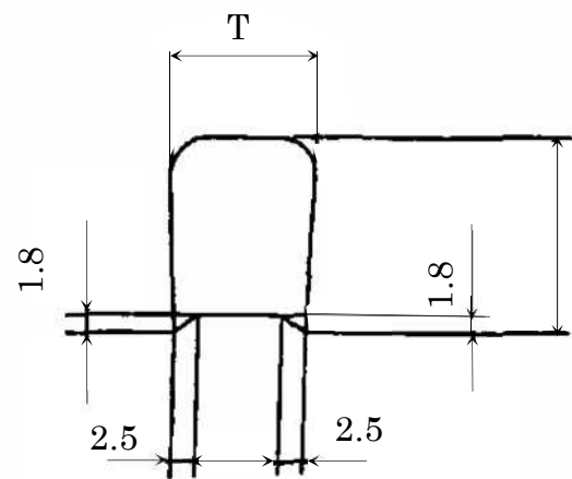
C-C 断面図
