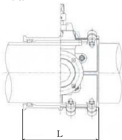
鑄鉄製割 T 字管 参考図 7 仮止水用仕切弁付割 T 字管
