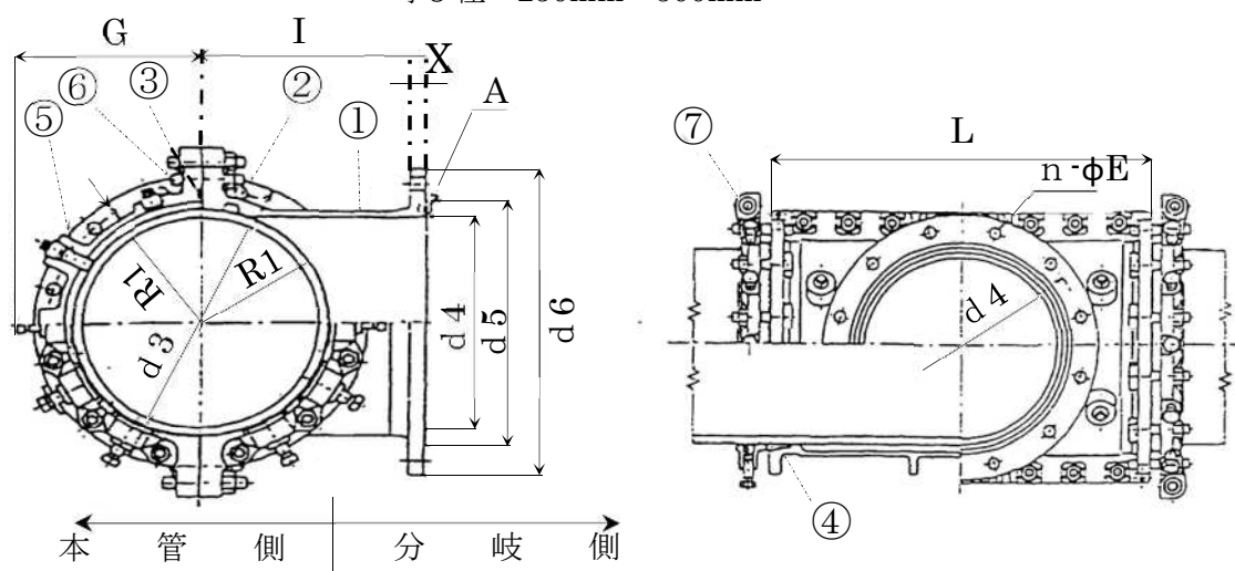
鑄鉄製割 T 字管 参考図 6 呼び径 250mm～500mm
