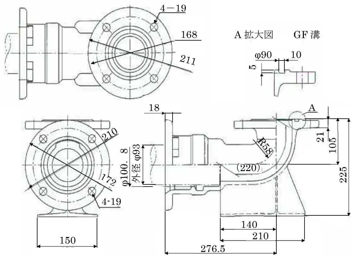
1. 2. 6 参考図1 (φ75×φ75)
