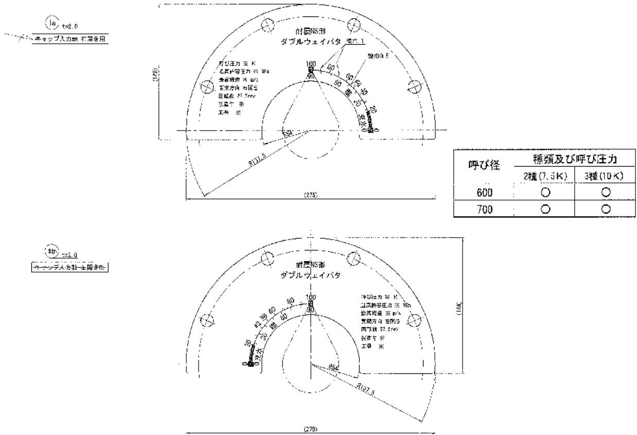
NS 形充水機能付バタフライ弁 参考図③-13 ( \phi 600 \cdot \phi 700 2種・3種併用 目盛板)
