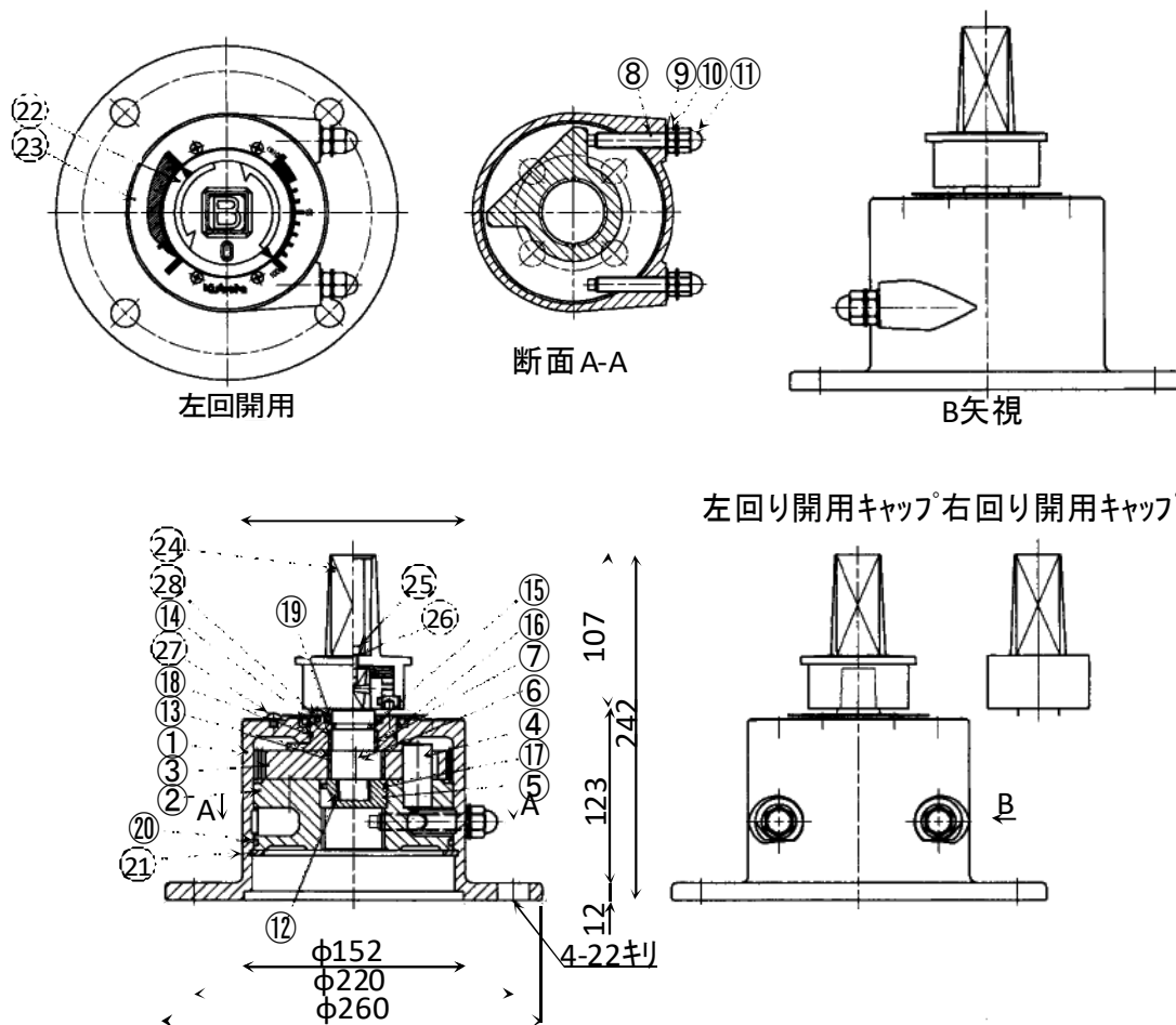
NS 形充水機能付バタフライ弁 参考図② (φ500)
