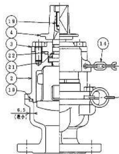
参考図 洗浄栓 2
