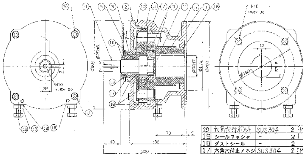
NS 形充水機能付バタフライ弁 参考図③－2 (\phi 500 操作機図)
