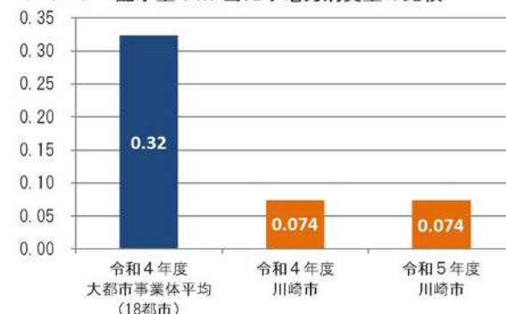
(kWh/m 3 ) 配水量 1 m 3 当たり電力消費量の比較
