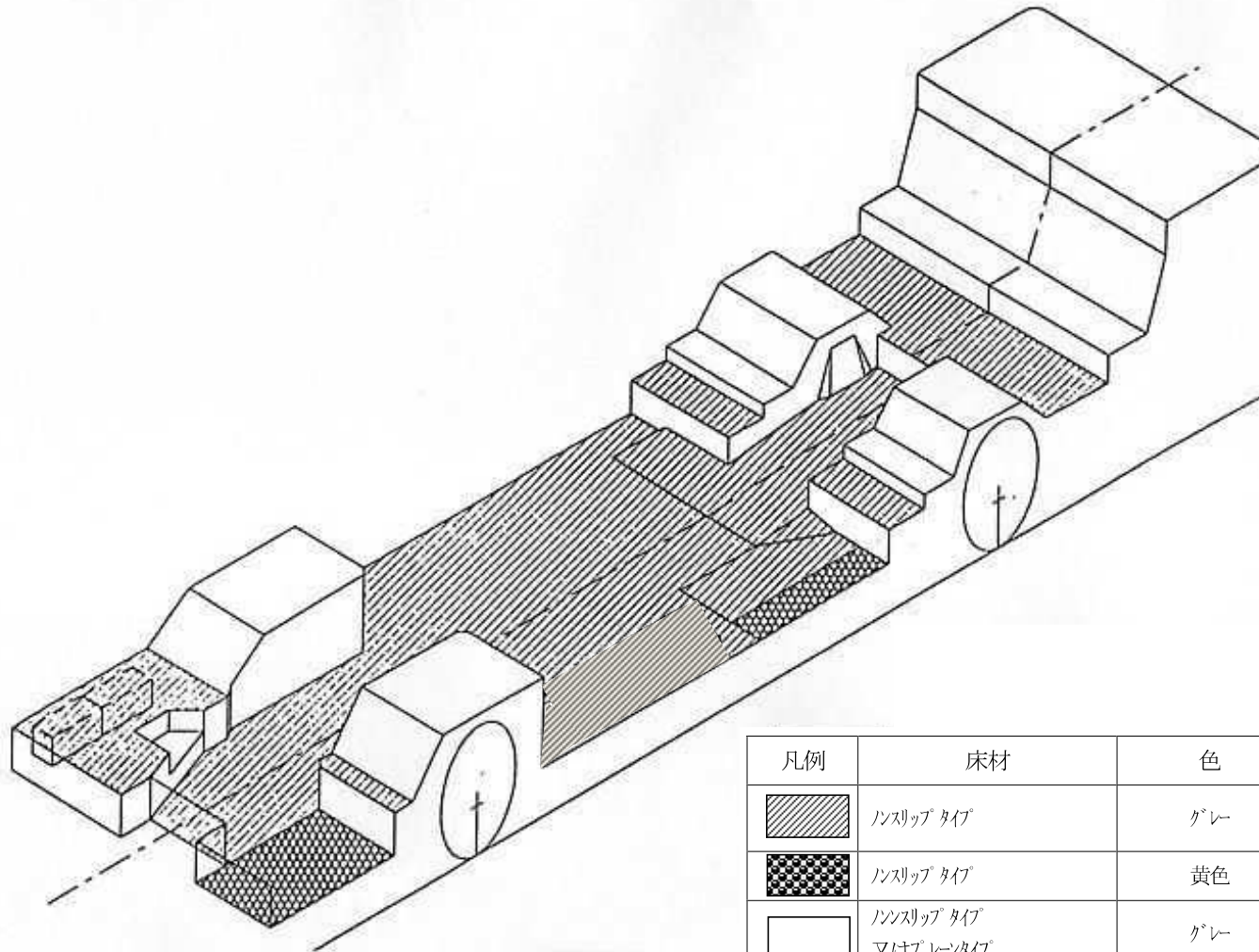
床上張材施工区分図
