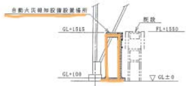
A~A 矢視 S=1/50
