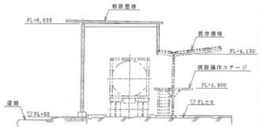
B~B 矢視 S=1/100
