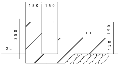
堰及び側溝詳細図 (S=1 / 200)
