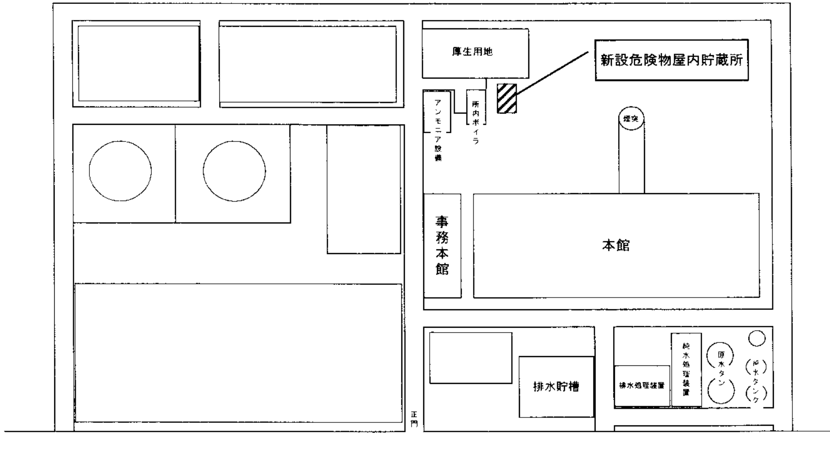
△△△事業所 構内配置図
