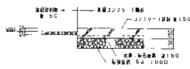
階段コンクリート鉄筋配筋断面図 S-1/200
