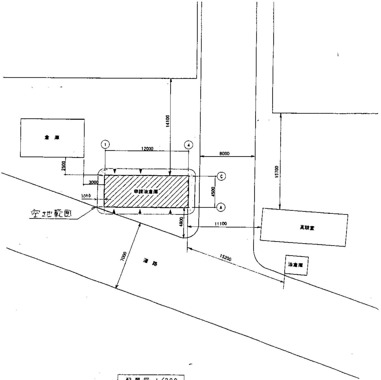
配置図 1/200
