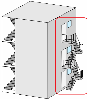
直通階段の増設
