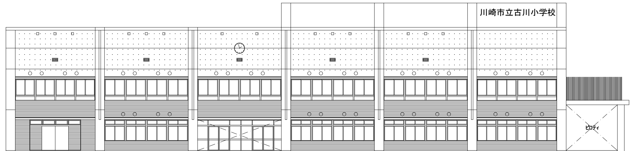
東側立面図
