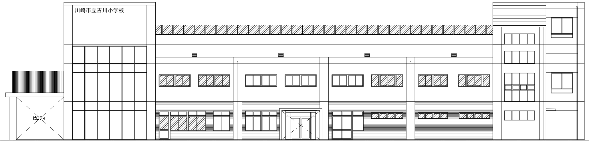
西側立面図
