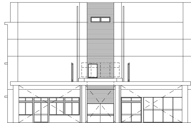
北側立面図
