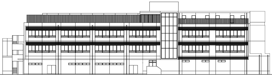
南側立面図
