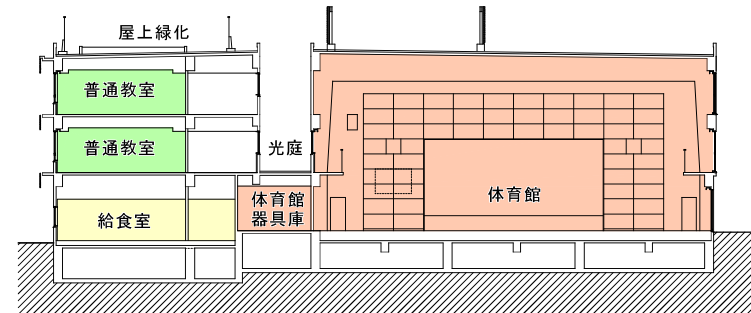
C-C' 断面図
