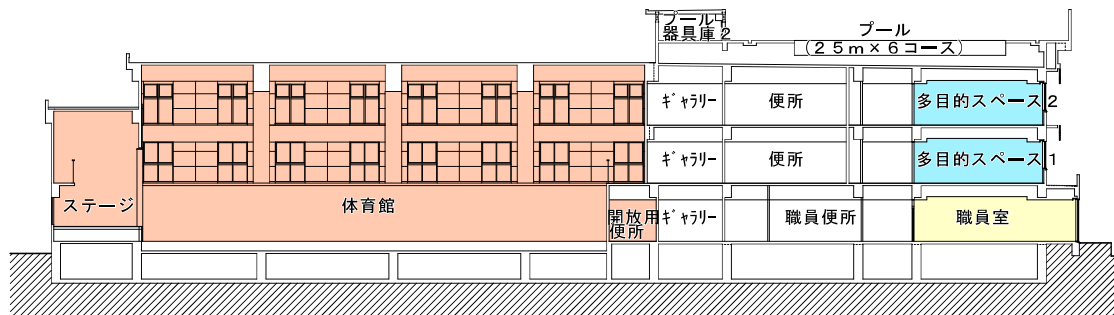
A-A' 断面図
