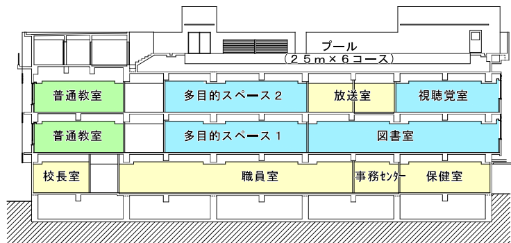
B-B' 断面図
