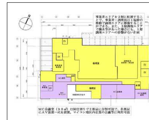
2階 平面図
