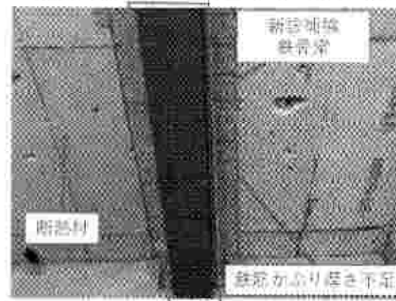
【④：5階天井スラブ下かぶり不足】
