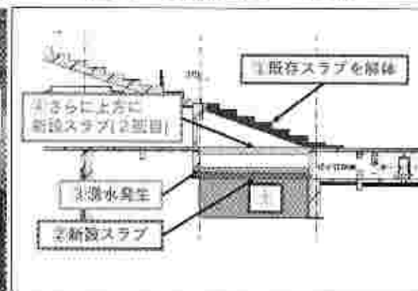
【大ホール断面イメージ図】
