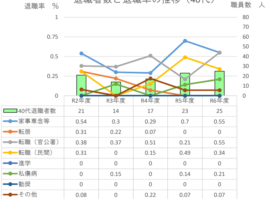
退職者数と退職率の推移（40代）
