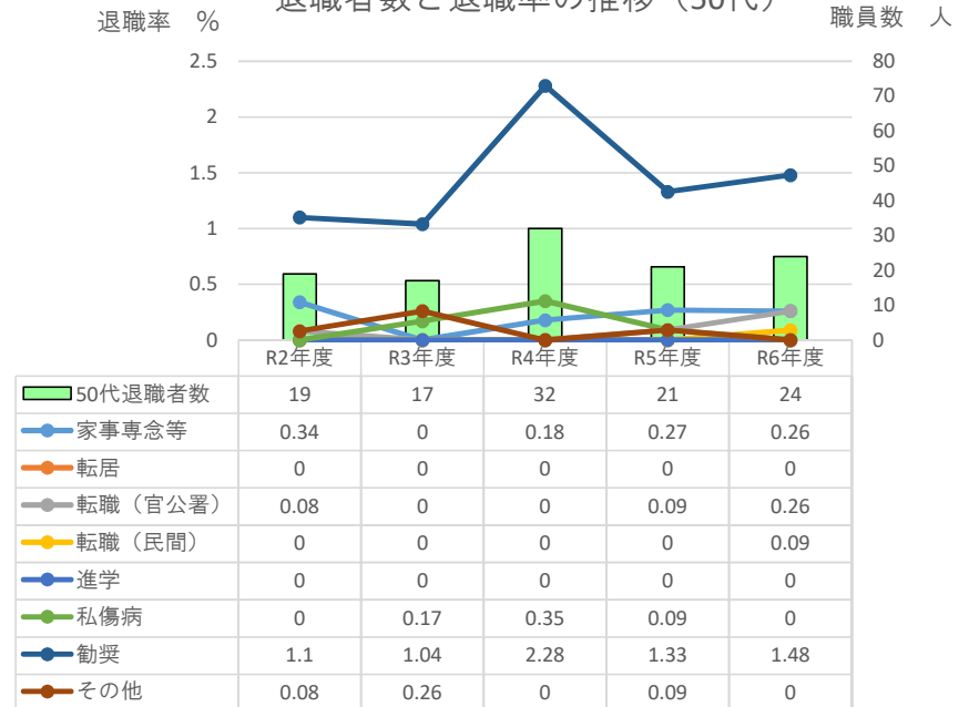
退職者数と退職率の推移（50代）
