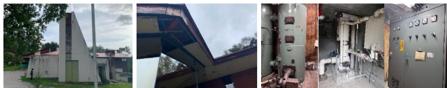
躯体の劣化が著しい エネルギー棟 渡り廊下軒裏の破損 ボイラー 消火設備 受変電設備 (耐用年数を越えた設備)
