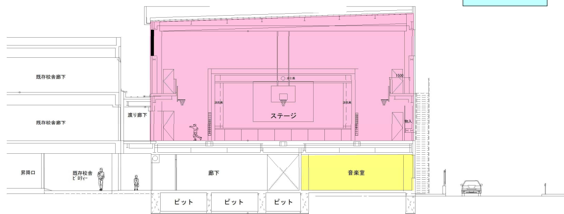
体育館棟 断面図②
