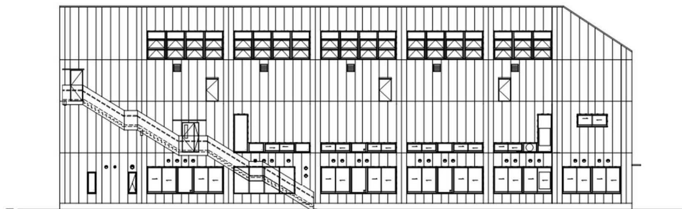
体育館棟 東立面図
