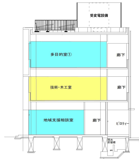
増築校舎棟 断面図①
