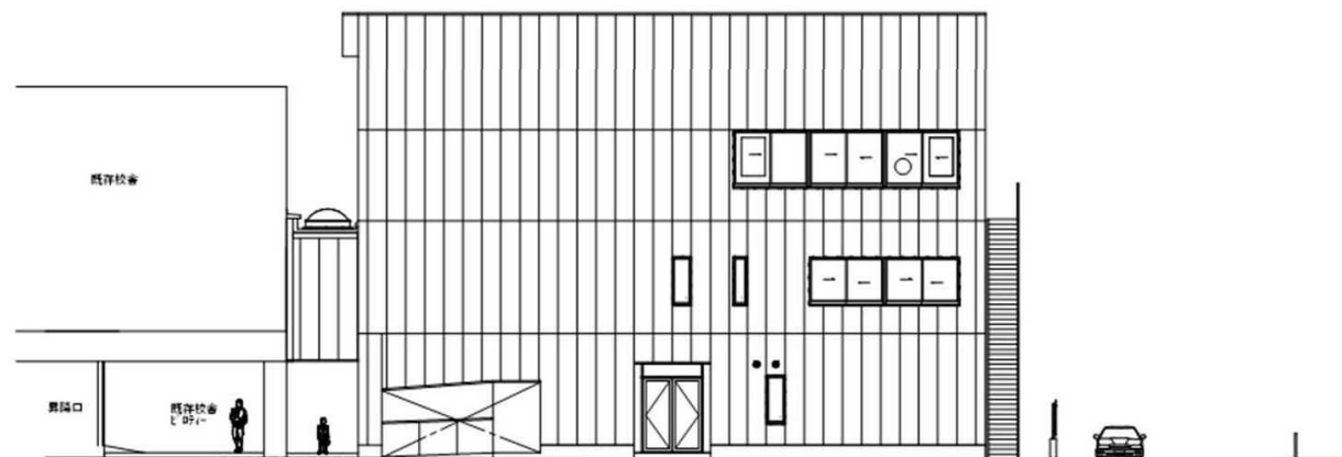
体育館棟 南立面図
