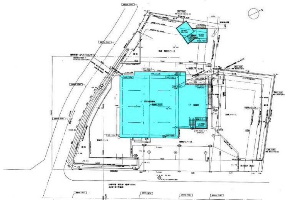
配置図
