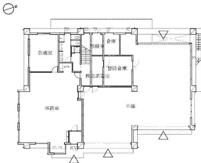
1F 平面図
