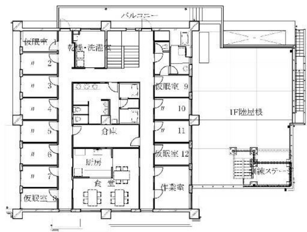
2F 平面図
